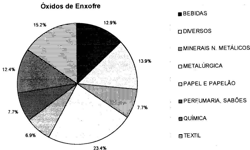
Gráfico 4 - Emissão de SO x por atividade industrial
