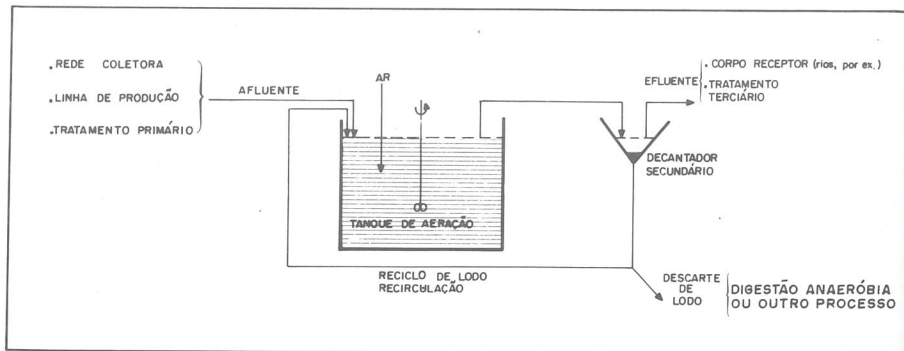
Figura 2 - Esquema do processo de lodos ativados.
