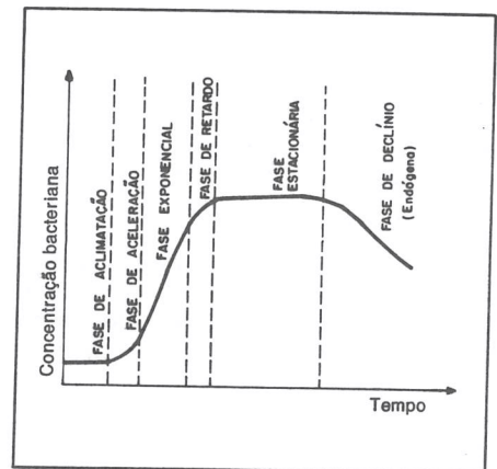
Figura 1 - Modelo de curva de crescimento de microrganismos em cultura pura.
