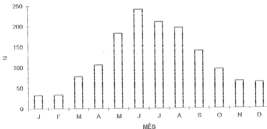
Figura 12: Monóxido de Carbono - Total de ultrapassagens do padrão por mês (1981 a 1994) - RMSP - Médias de 8h.
