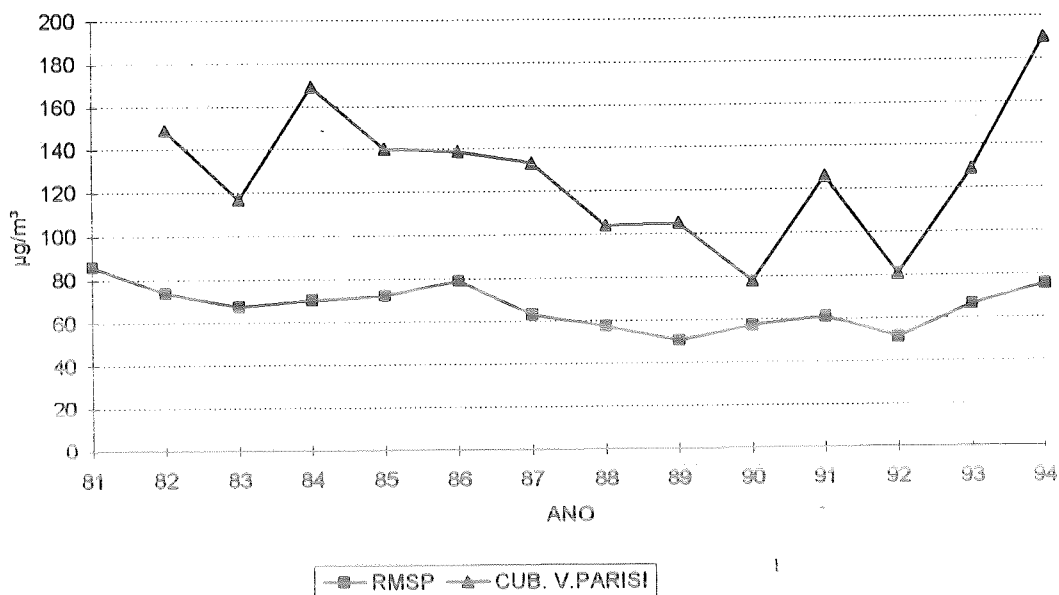
Figura 9: Partículas Inaláveis - Evolução das concentrações médias anuais na RMSP e Cubatão - Vila Parisi.
