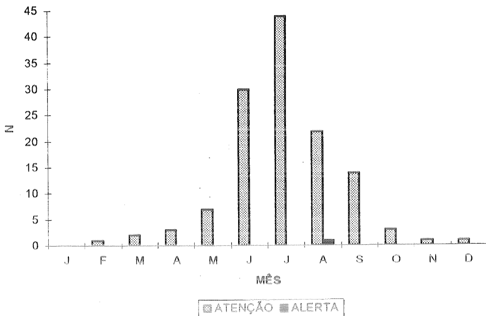
Figura 13: Monóxido de Carbono - Total de ultrapassagens de níveis críticos por mês (1981 a 1994) - RMSP - Médias de 8h.
