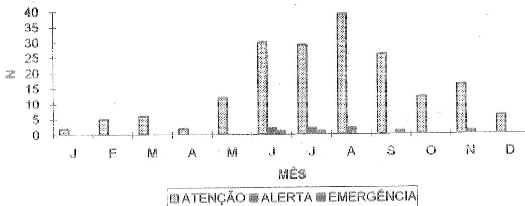
Figura 8: Partículas Inaláveis - Total de ultrapassagens de níveis críticos por mês (1982 a 1994) - Cubatão - Vila Parisi
