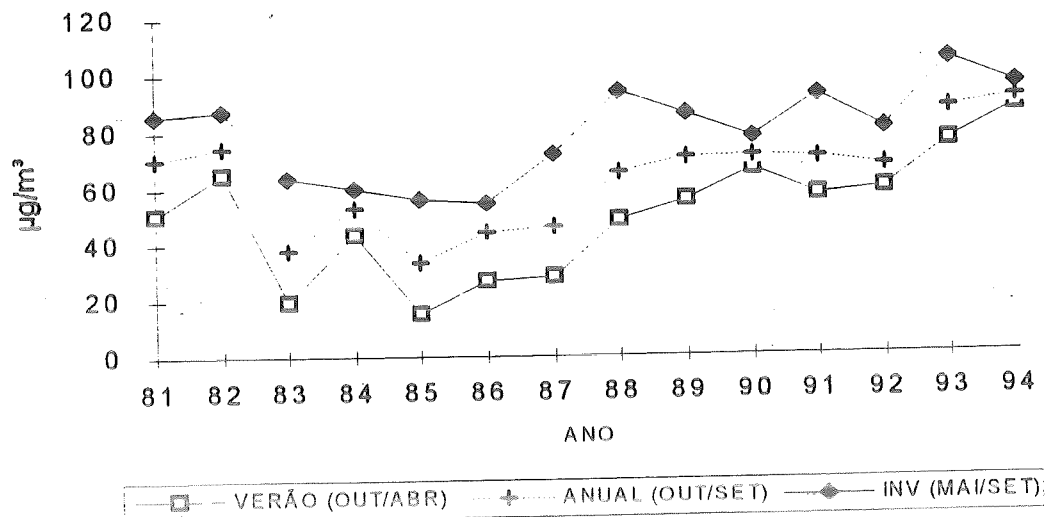
Figura 2: Partículas Inaláveis - Osasco (1981 a 1994)
