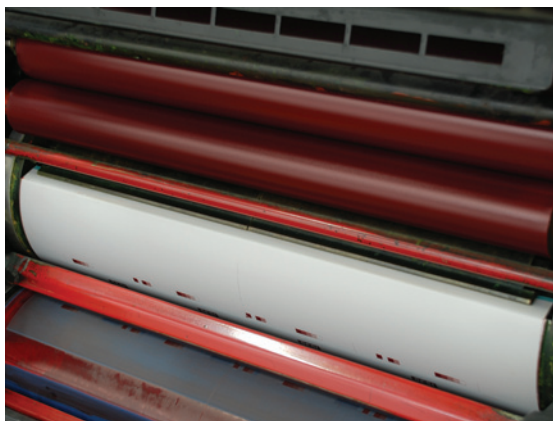
Figura 5 - Impressora offset – Detalhe dos cilindros porta-chapa e entintador de uma máquina de impressão.
