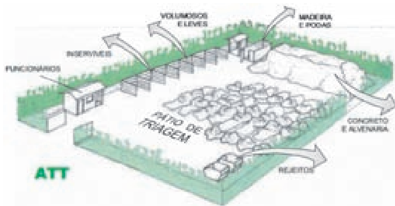
FIGURA 04. Exemplo de layout de uma ATT
