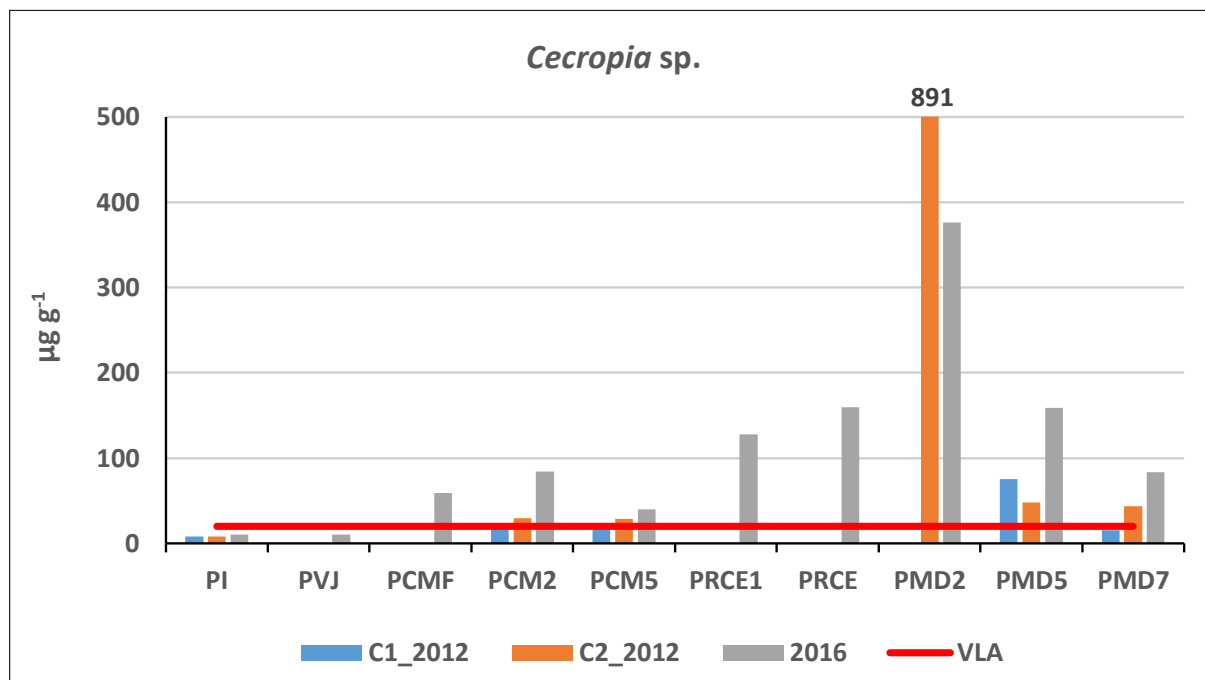
Gráfico 4.3.3 – Concentração foliar de fluoreto para Cecropia sp. (Embaúba) coletadas em 2012 e 2016
