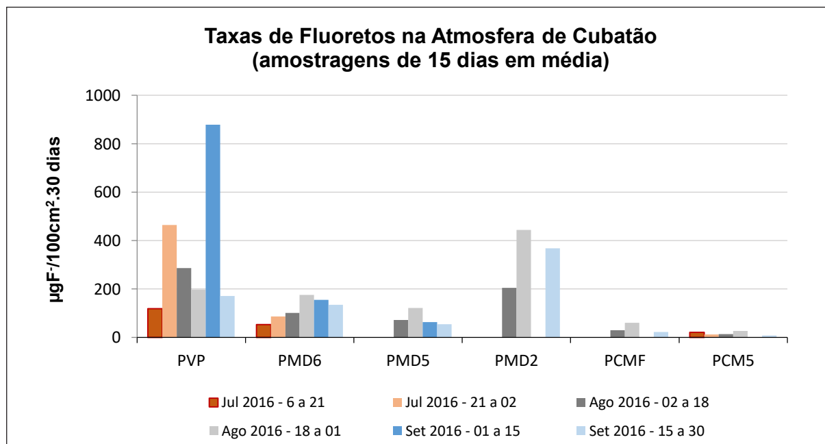
Gráfico 4.1.1 – Taxas de fluoretos medidas no período de 06/07 a 30/09, por ponto de amostragem, no Município de Cubatão
