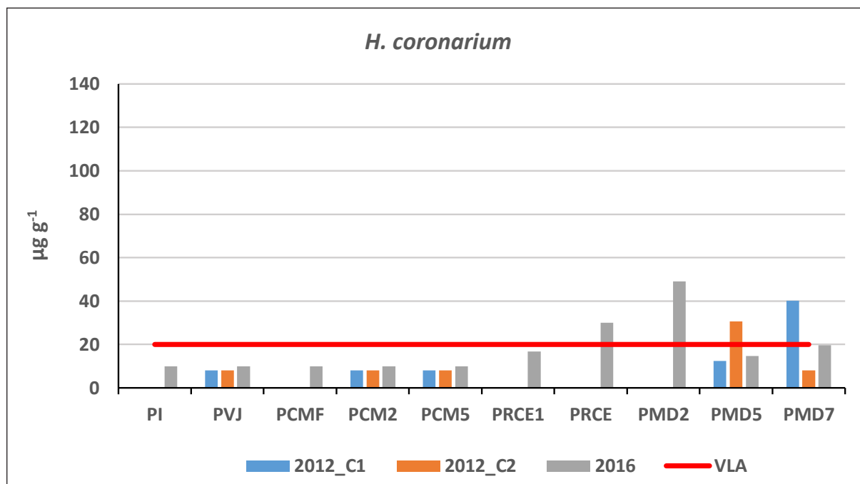
Gráfico 4.3.4 – Concentração foliar de fluoreto para H. coronarium (Lírio-do-brejo) coletadas em 2012 e 2016
