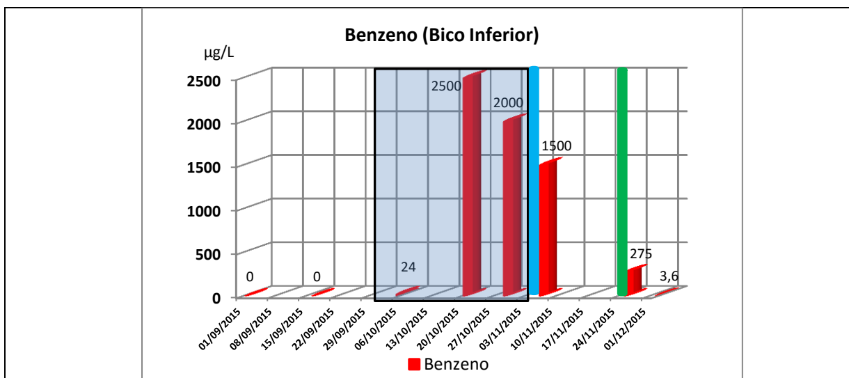
Gráfico 4.2 - Evolução das concentrações de Benzeno em amostras de água coletadas na parte inferior da coluna.
