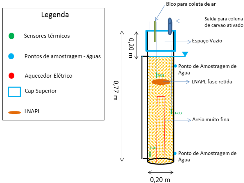
Figura 3-3 – Esquema de Montagem da Coluna de Ensaio.
