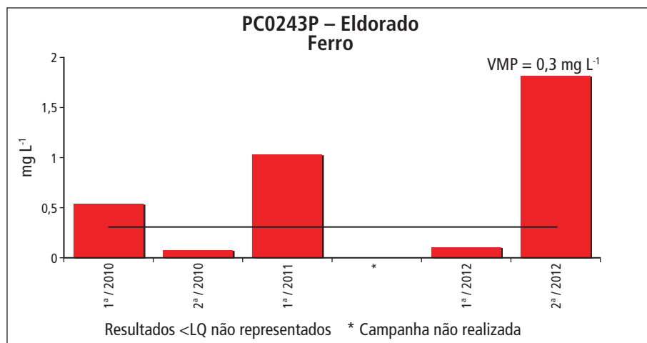
Gráfico 5.8.1 – Série histórica das concentrações de ferro no ponto PC0243P – Eldorado, Aquífero Pré-Cambriano
