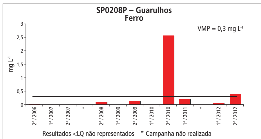
Gráfico 5.4.16 – Série histórica das concentrações de ferro no ponto SP0208P – Guarulhos, Aquífero São Paulo
