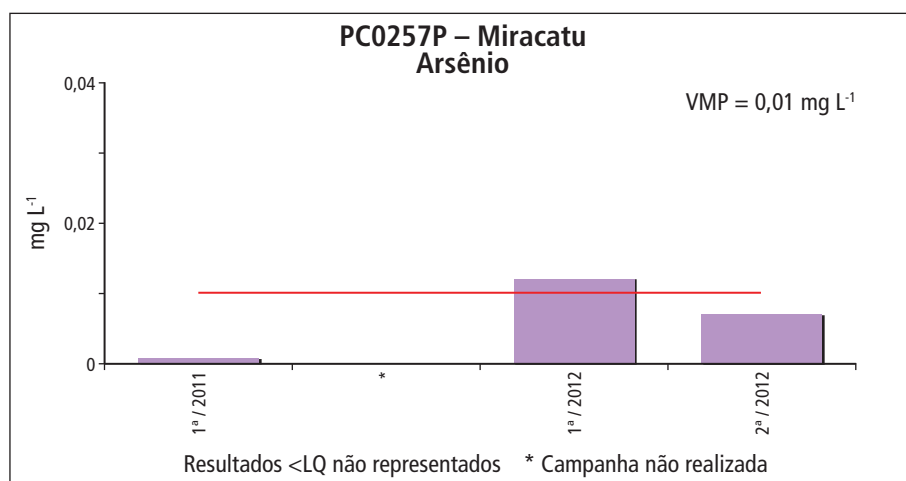
Gráfico 5.8.2 – Série histórica das concentrações de arsênio no ponto PC0257P – Miracatu, Aquífero Pré-Cambriano
