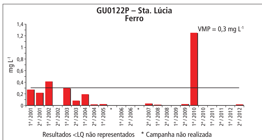
Gráfico 5.6.1 – Série histórica das concentrações de ferro no ponto GU0122P – Santa Lúcia, Aquífero Guarani
