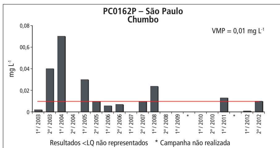
Gráfico 5.4.9 – Série histórica das concentrações de chumbo no ponto PC0162P –São Paulo, Aquífero Pré-Cambriano
