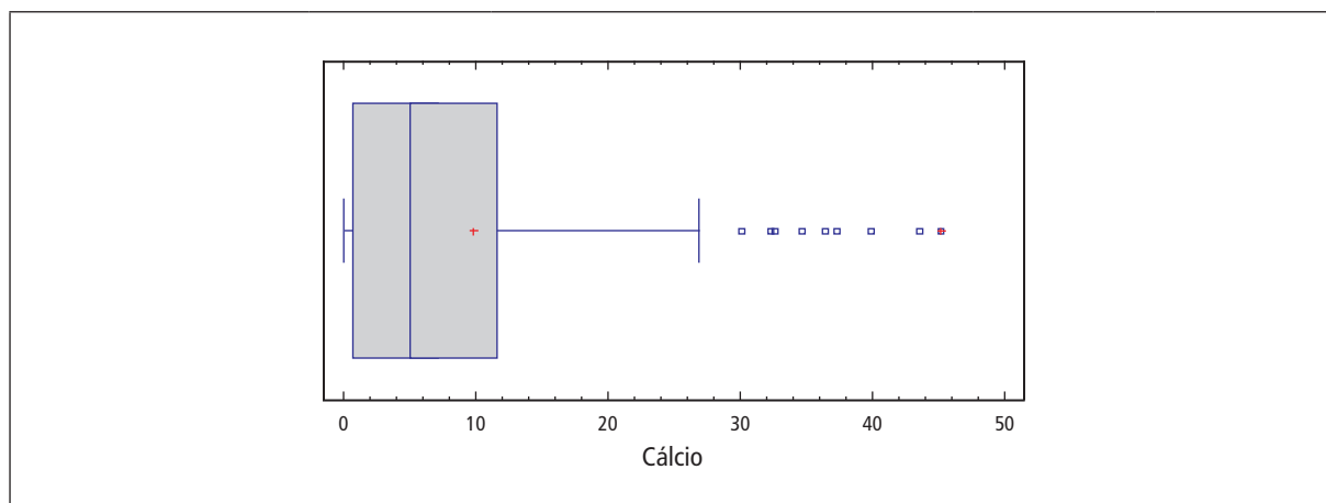
Gráfico 6.3 – Boxplot das concentrações de Cálcio ( \text{mg L}^{-1} ) das amostras de água subterrânea do Aquífero Bauru no período de 2010 a 2012
