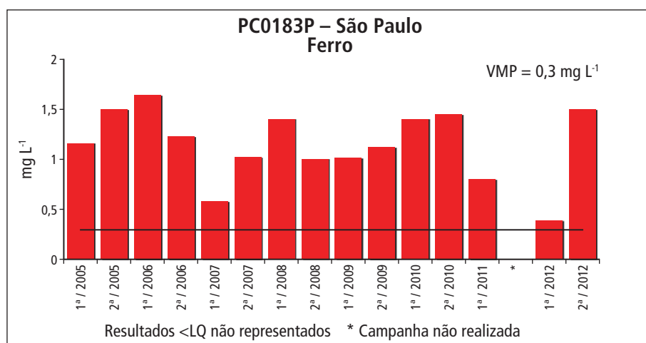
Gráfico 5.4.12 – Série histórica das concentrações de ferro no ponto PC0183P – São Paulo, Aquífero Pré-Cambriano
