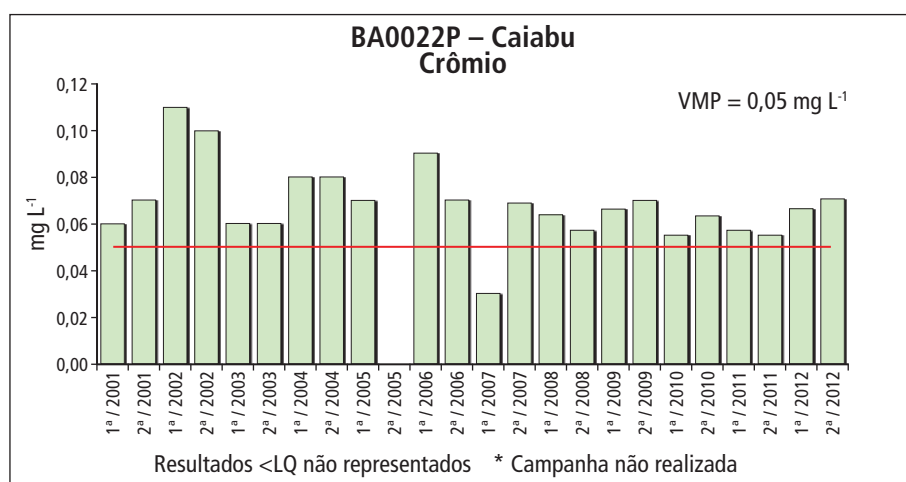
Gráfico 5.18.2 – Série histórica das concentrações de cromo no ponto BA0022P – Caiabu, Aquífero Bauru
