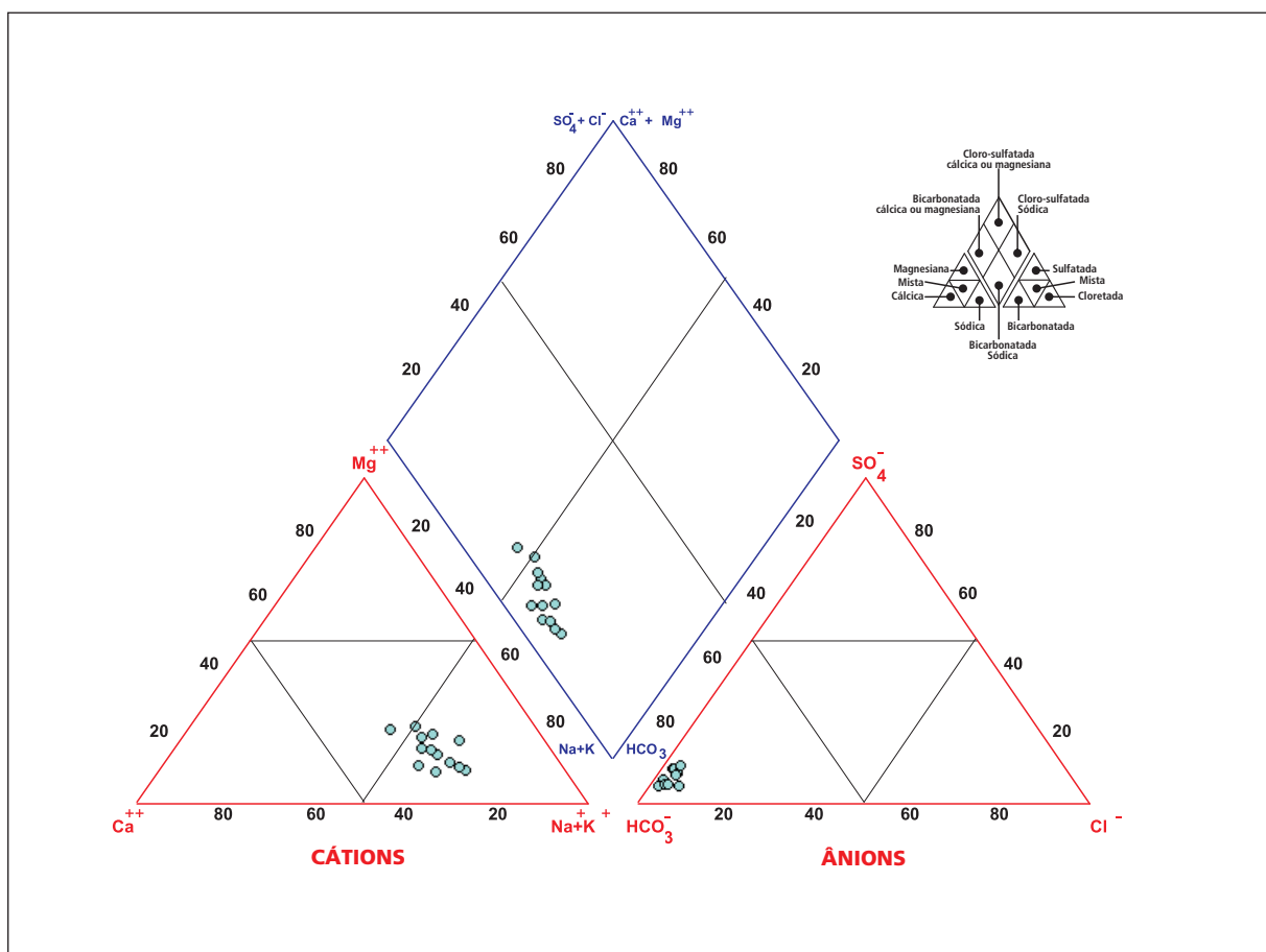
Figura 4.7.1 – Classificação das águas subterrâneas do Aquífero São Paulo, segundo o Diagrama de Piper
