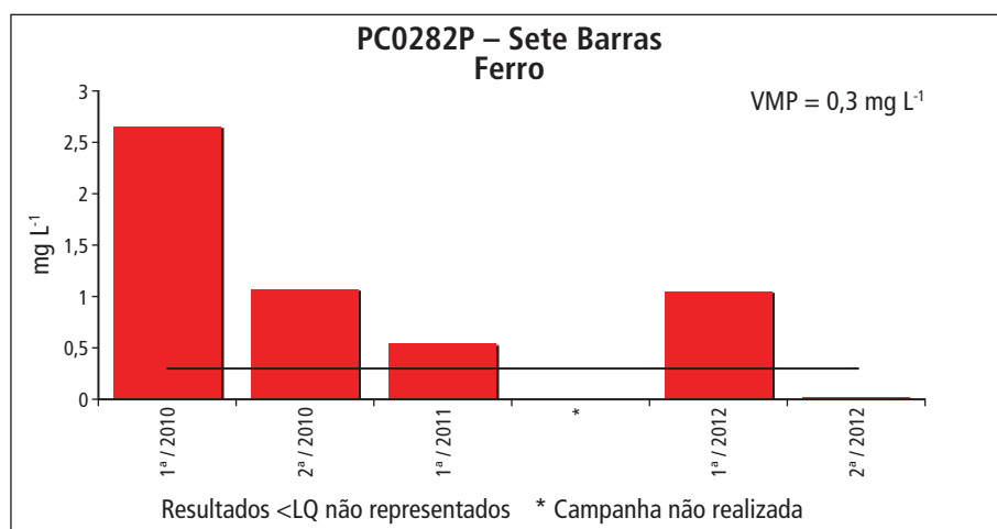
Gráfico 5.8.5 – Série histórica das concentrações de ferro no ponto PC0282P – Sete Barras, Aquífero Pré-Cambriano
