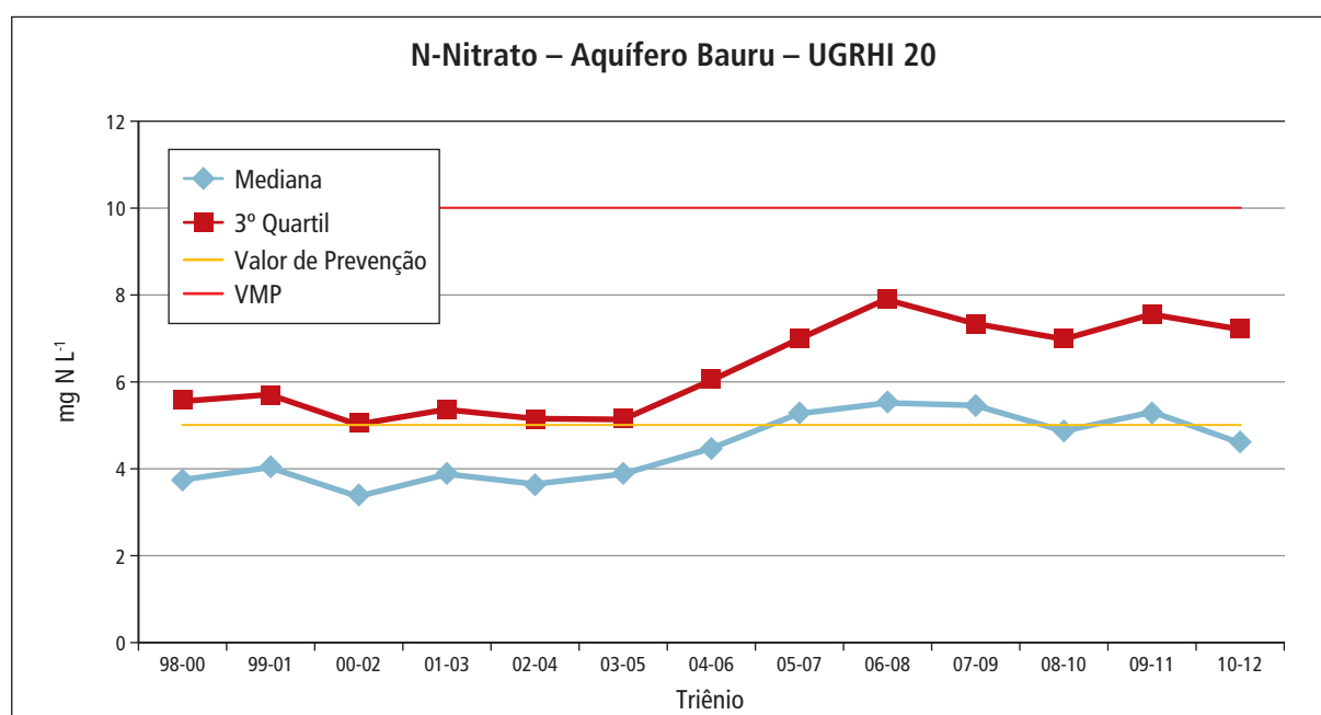
Gráfico 5.17.5 – Tendência das concentrações de nitrato no Aquífero Bauru – UGRHI 20
