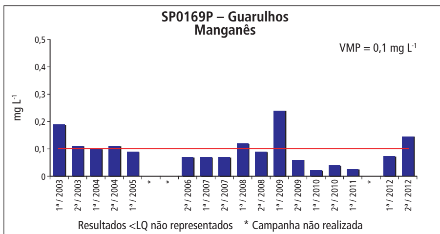
Gráfico 5.4.15 – Série histórica das concentrações de manganês no ponto SP0169P – Guarulhos, Aquífero São Paulo
