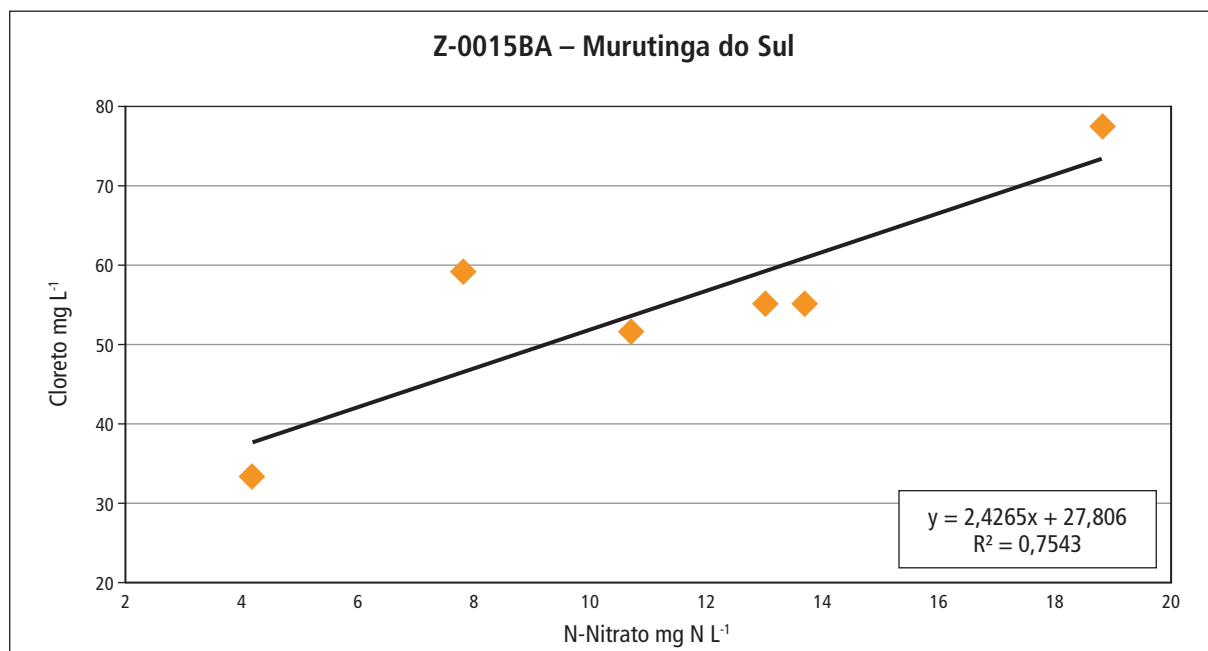
Gráfico 6.6 – Correlação entre Nitrato e Cloreto nas amostras de água subterrânea do ponto de Murutinga do Sul no período de 2010 a 2012
