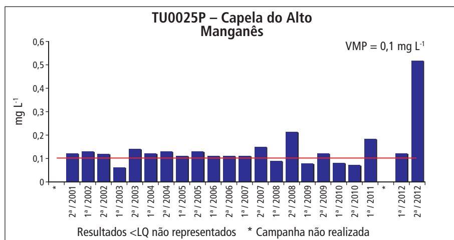
Gráfico 5.7.3 – Série histórica das concentrações de manganês no ponto TU0025P – Capela do Alto, Aquífero Tubarão
