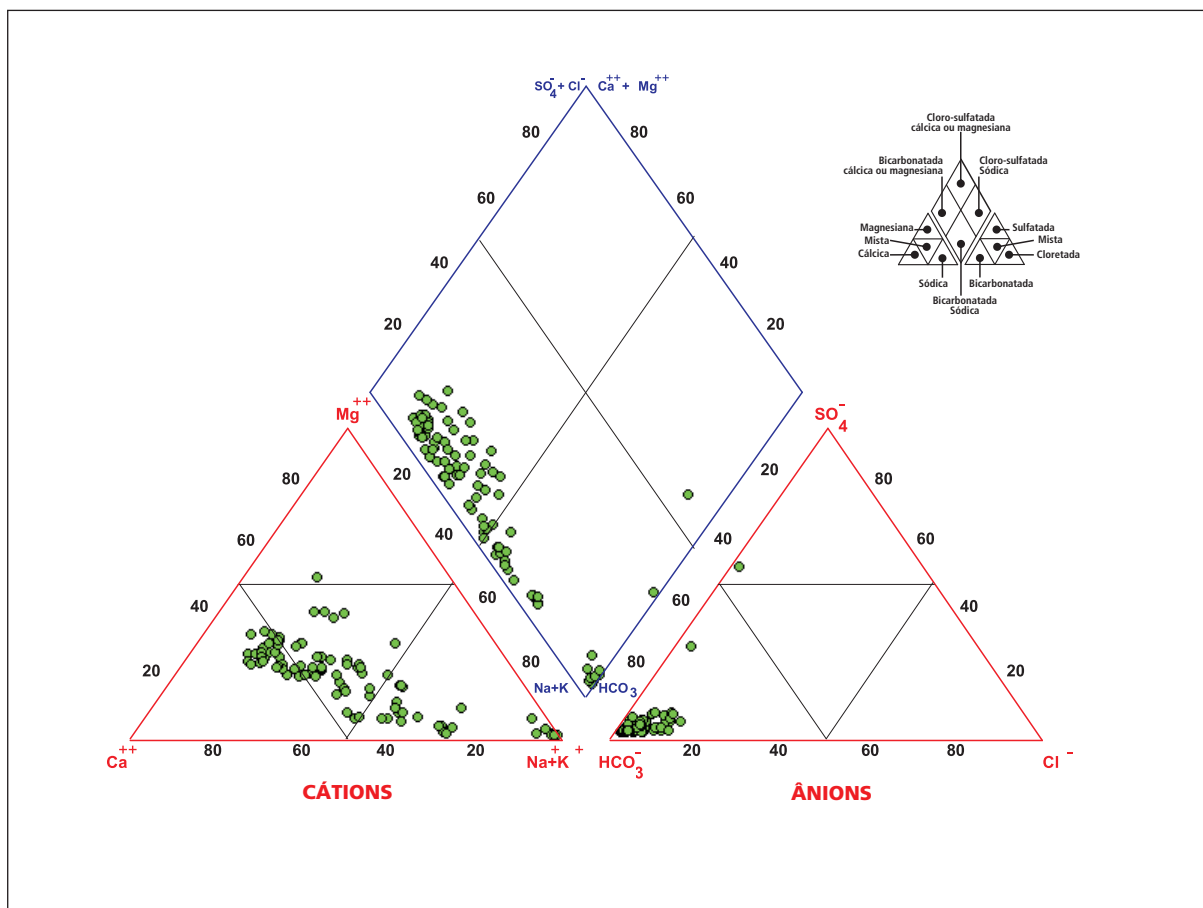
Figura 4.2.1 – Classificação das águas do Aquífero Serra Geral, segundo o Diagrama de Piper
