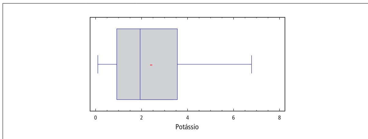
Gráfico 6.10 – Boxplot das concentrações de Potássio ( \text{mg L}^{-1} ) das amostras de água subterrânea do Aquífero Guarani no período de 2010 a 2012
