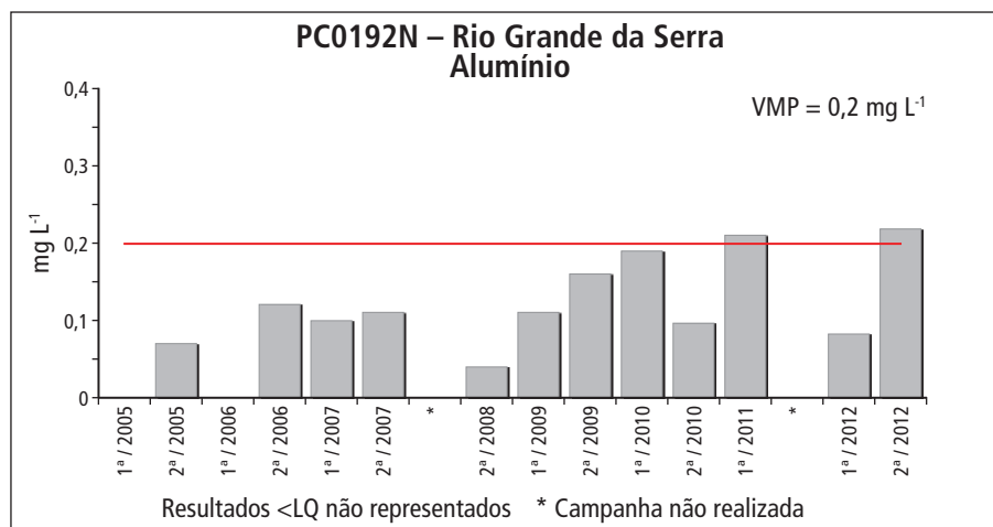
Gráfico 5.4.5 – Série histórica das concentrações de alumínio no ponto PC0192N – Rio Grande da Serra, Aquífero Pré-Cambriano
