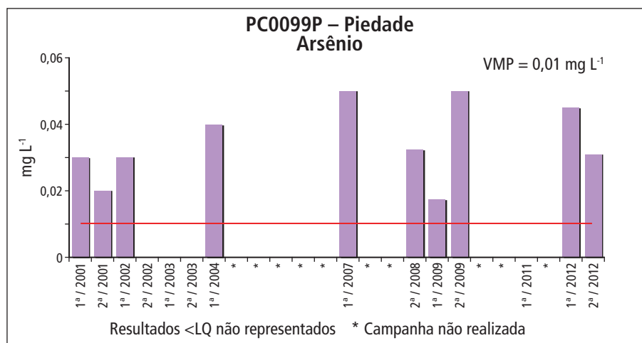
Gráfico 5.7.1 – Série histórica das concentrações de arsênio no ponto PC0099P – Piedade, Aquífero Pré-Cambriano
