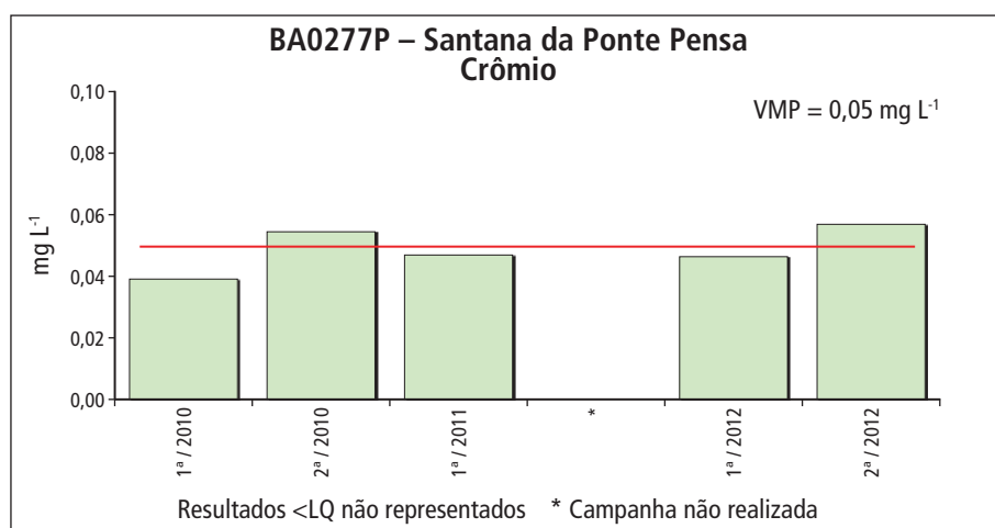
Gráfico 5.15.6 – Série histórica das concentrações de cromo no ponto BA0277P – Santana da Ponte Pensa, Aquífero Bauru
