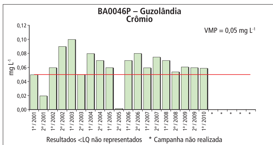
Gráfico 5.15.3 – Série histórica das concentrações de cromo no ponto BA0046P – Guzolândia, Aquífero Bauru
