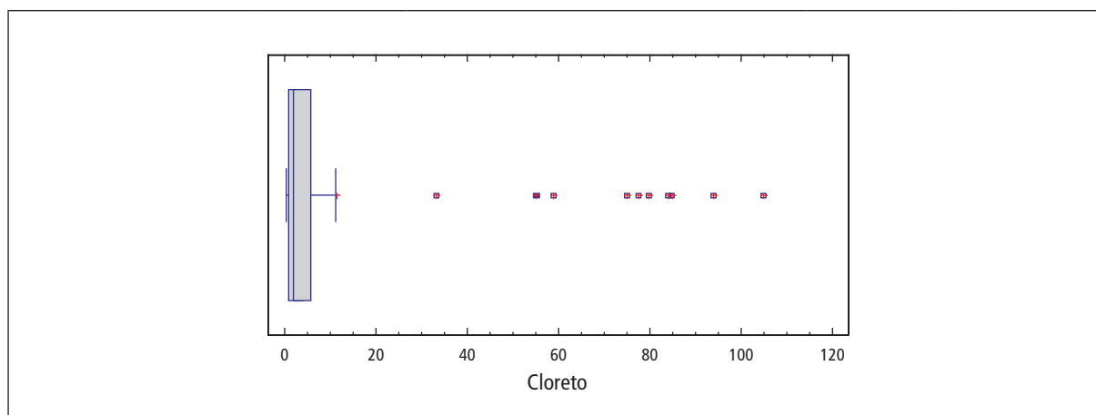
Gráfico 6.2 – Boxplot das concentrações de Cloreto ( \text{mg L}^{-1} ) das amostras de água subterrânea do Aquífero Bauru no período de 2010 a 2012
