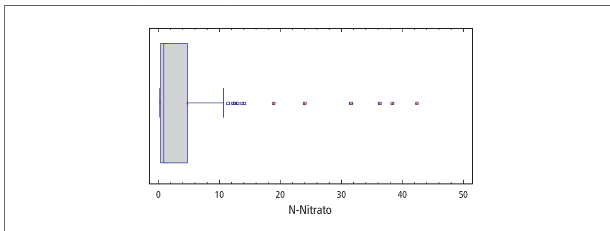
Gráfico 6.1 – Boxplot das concentrações de Nitrato ( \text{mg N L}^{-1} ) das amostras de água subterrânea do Aquífero Bauru no período de 2010 a 2012
