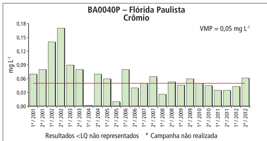
Gráfico 5.18.3 – Série histórica das concentrações de cromo no ponto BA0040P – Flórida Paulista, Aquífero Bauru
