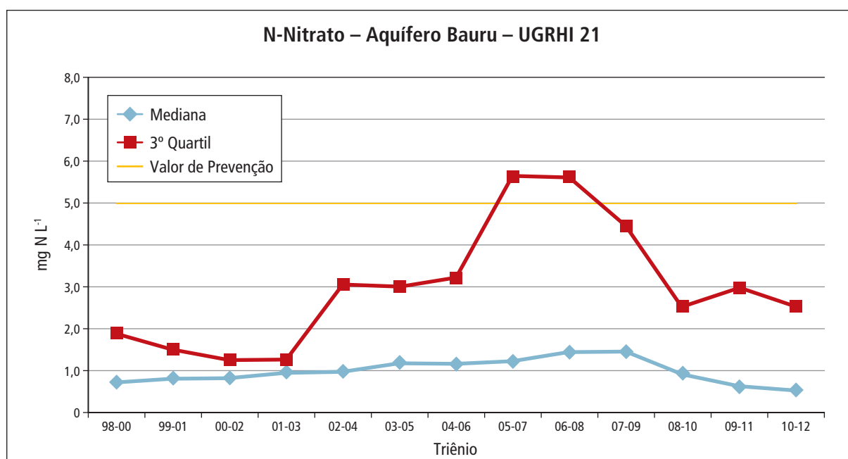
Gráfico 5.18.7 – Tendência das concentrações de nitrato no Aquífero Bauru – UGRHI 21
