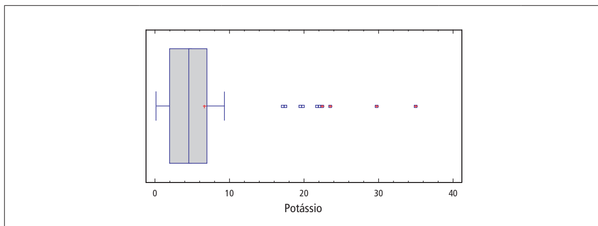
Gráfico 6.4 – Boxplot das concentrações de Potássio ( \text{mg L}^{-1} ) das amostras de água subterrânea do Aquífero Bauru no período de 2010 a 2012
