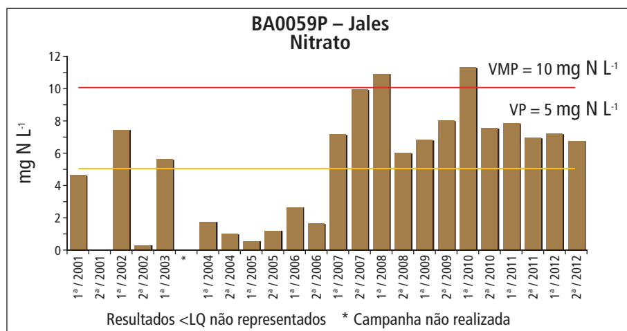
Gráfico 5.15.4 – Série histórica das concentrações de nitrato no ponto BA0059P – Jales, Aquífero Bauru
