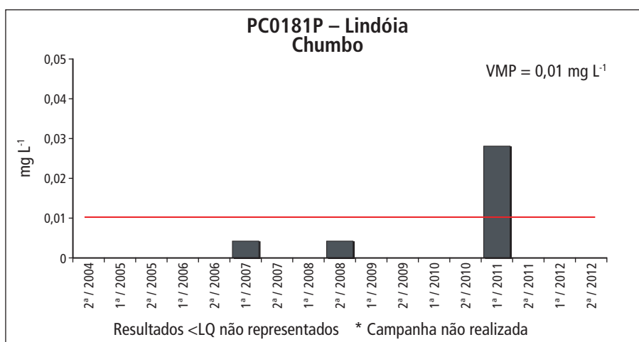
Gráfico 5.6.4 – Série histórica das concentrações de chumbo no ponto PC0181P – Lindóia, Aquífero Pré-Cambriano
