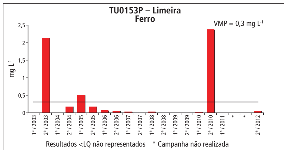
Gráfico 5.3.10 – Série histórica dos resultados para ferro no ponto TU0153P – Limeira, Aquífero Tubarão
