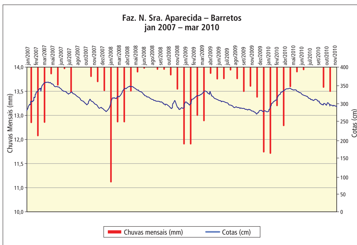
Gráfico 6.13 – Variação do aquífero freático em Barretos em função da pluviometria
