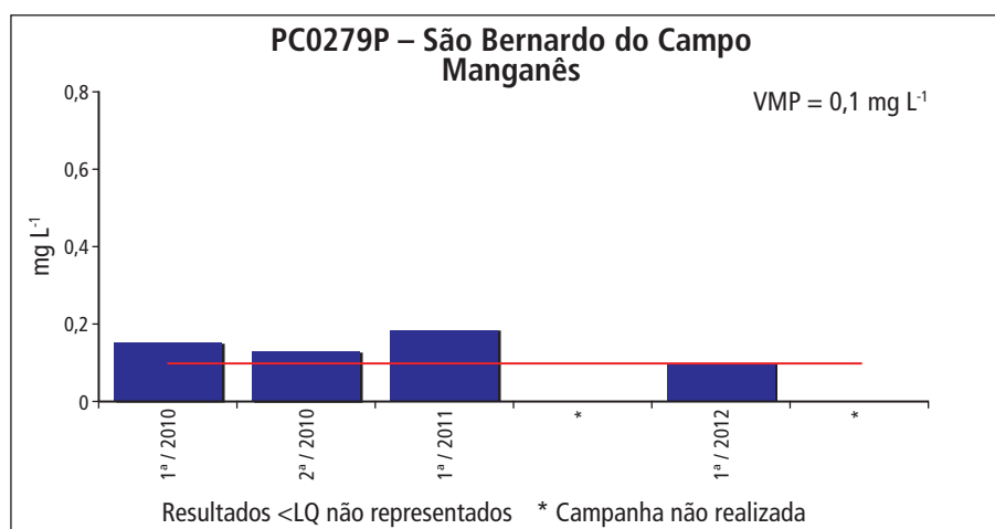
Gráfico 5.4.7 – Série histórica das concentrações de manganês no ponto PC0279P – S. Bernardo do Campo, Aquífero Pré-Cambriano
