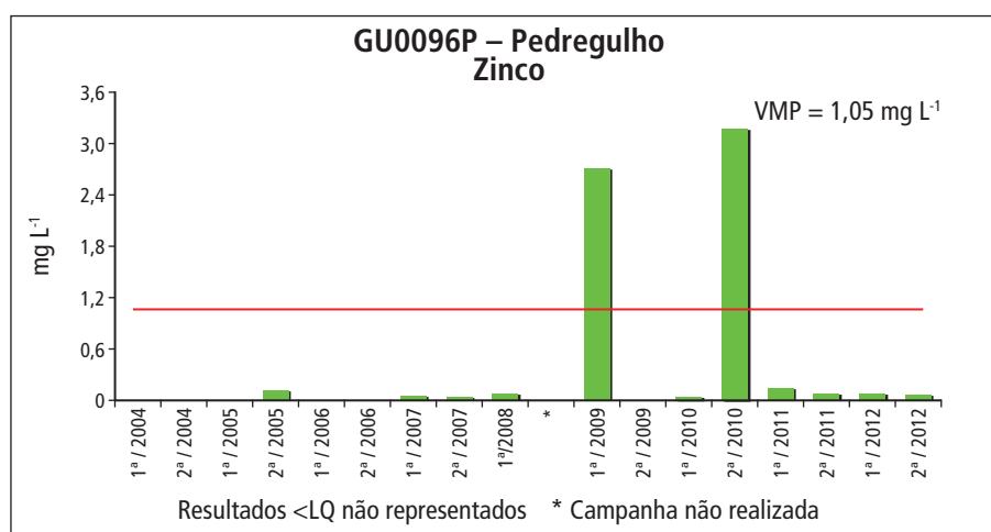
Gráfico 5.5.1 – Série histórica das concentrações de zinco no ponto GU0096P – Pedregulho, Aquífero Guarani
