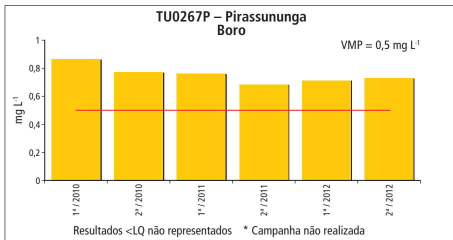
Gráfico 5.6.6 – Série histórica das concentrações de boro no ponto TU0267P – Pirassununga, Aquífero Tubarão
