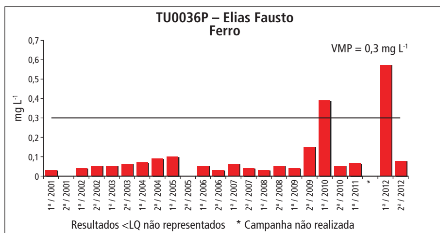
Gráfico 5.3.5 – Série histórica das concentrações de ferro no ponto TU0036P – Elias Fausto, Aquífero Tubarão
