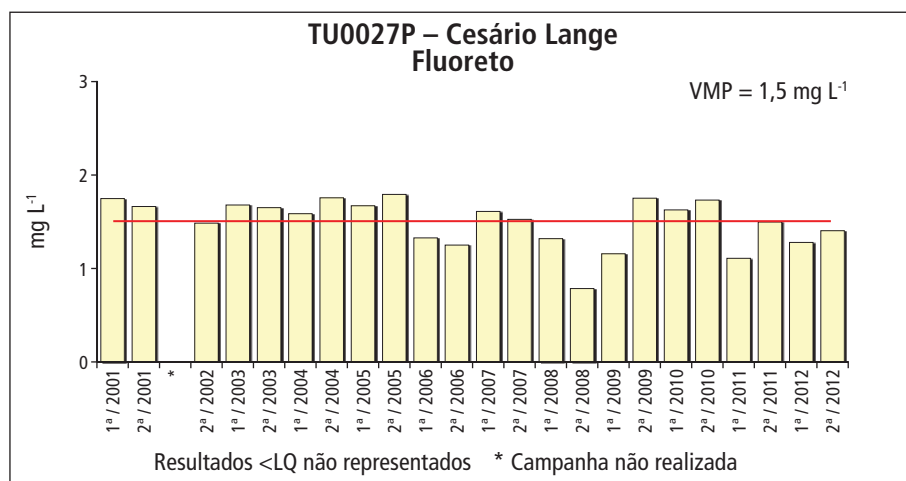
Gráfico 5.7.4 – Série histórica das concentrações de fluoreto no ponto TU0027P – Cesário Lange, Aquífero Tubarão
