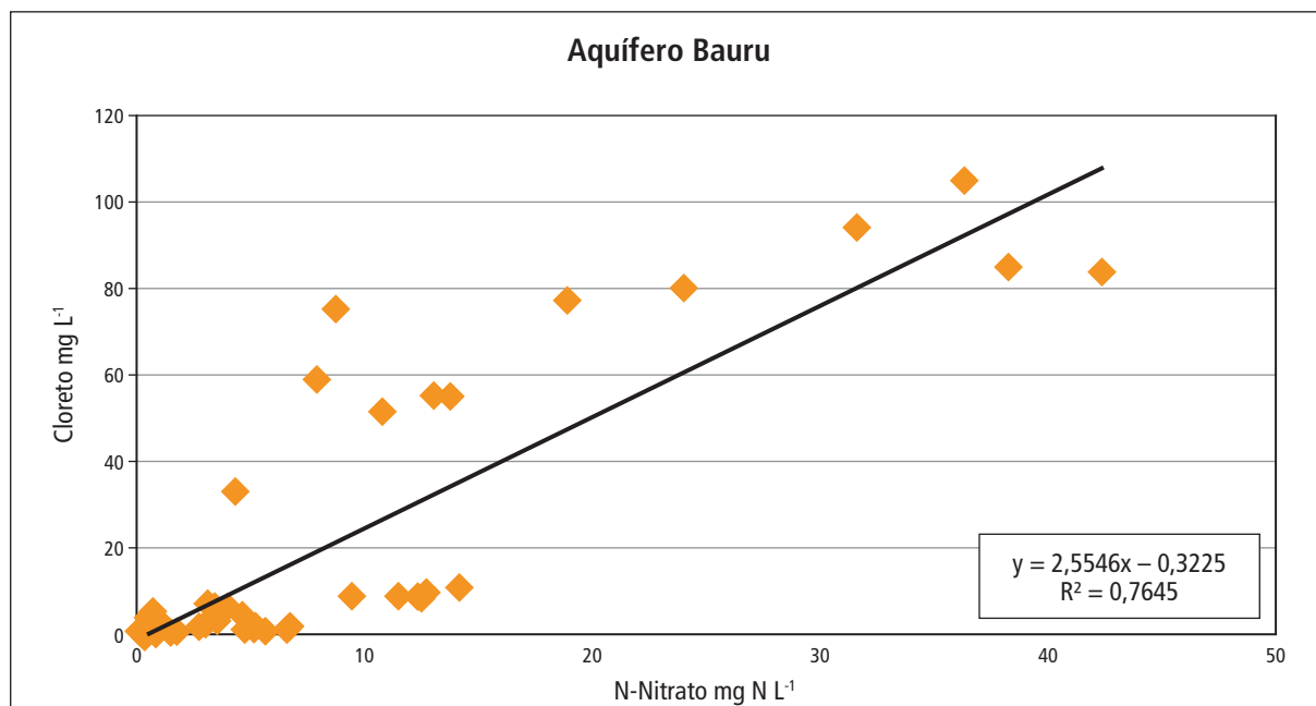
Gráfico 6.5 – Correlação entre Nitrato e Cloreto nas amostras de água subterrânea do Aquífero Bauru no período de 2010 a 2012
