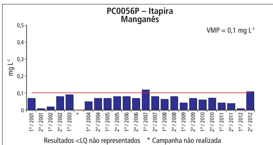
Gráfico 5.6.3 – Série histórica das concentrações de manganês no ponto PC0056P – Itapira, Aquífero Pré-Cambriano
