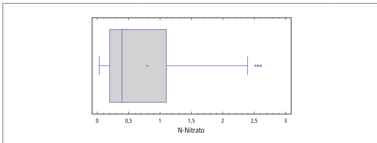
Gráfico 6.7 – Boxplot das concentrações de Nitrato ( \text{mg N L}^{-1} ) das amostras de água subterrânea do Aquífero Guarani no período de 2010 a 2012
