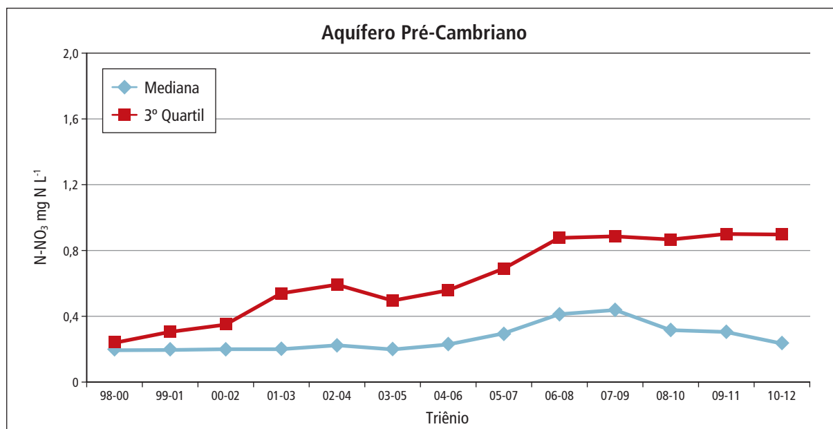
Gráfico 7.2.3 – Tendência das concentrações de nitrato no Aquífero Pré-Cambriano, no período de 1998 a 2012
