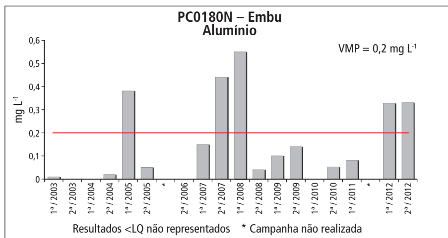
Gráfico 5.4.4 – Série histórica das concentrações de alumínio no ponto PC0180N – Embu, Aquífero Pré-Cambriano
