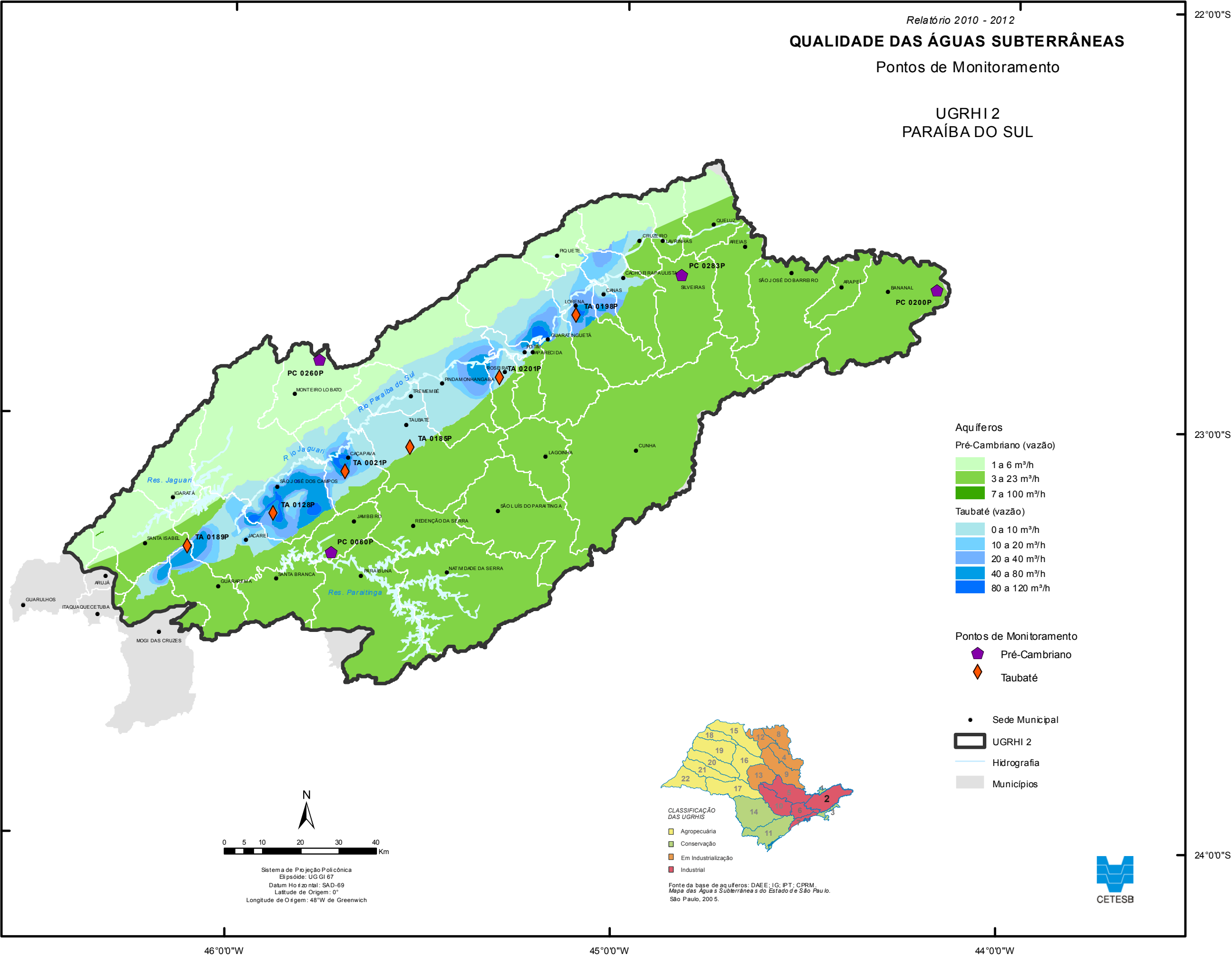
Figura 5.1.1 – Localização dos pontos de monitoramento da UGRHI 2 – Paraíba do Sul
