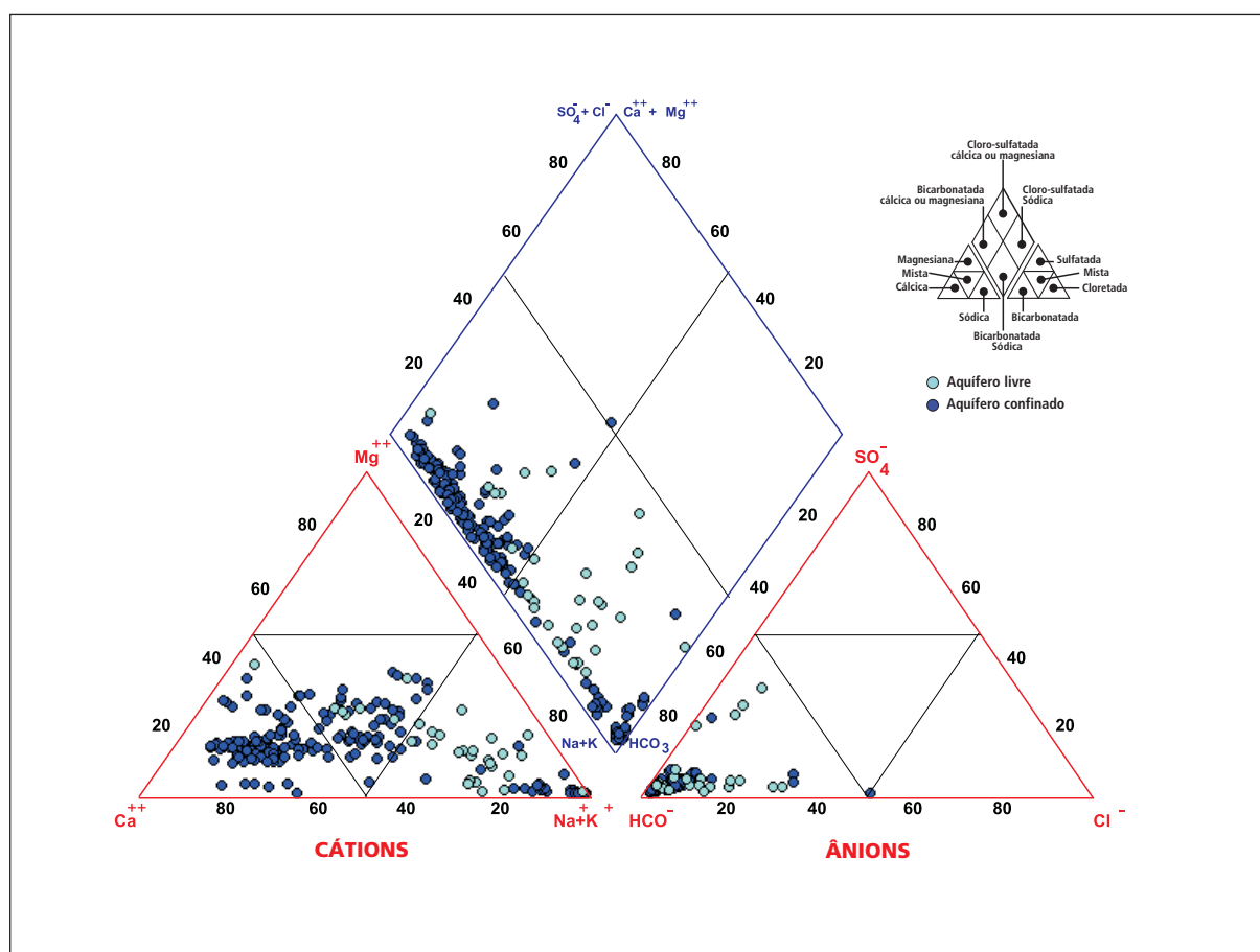
Figura 4.3.1 – Classificação das águas do Aquífero Guarani, segundo o Diagrama de Piper
