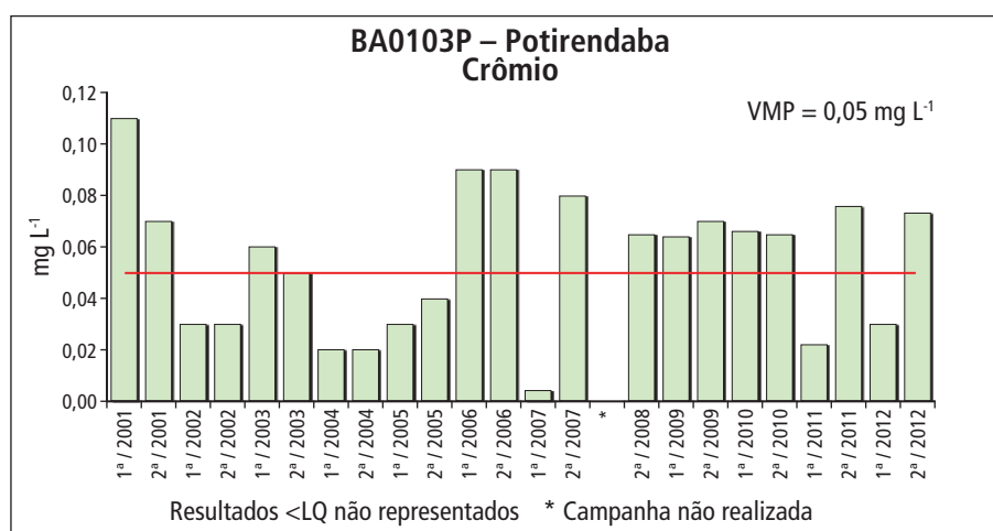
Gráfico 5.13.1 – Série histórica das concentrações de crômio no ponto BA0103P – Potirendaba, Aquífero Bauru
