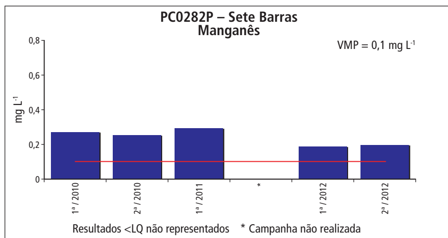
Gráfico 5.8.6 – Série histórica das concentrações de manganês no ponto PC0282P – Sete Barras, Aquífero Pré-Cambriano
