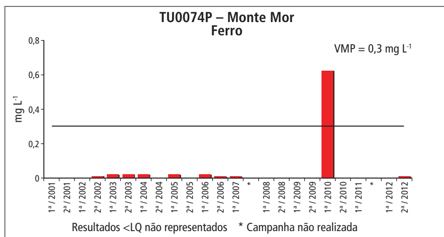
Gráfico 5.3.11 – Série histórica das concentrações de ferro no ponto TU0074P – Monte Mor, Aquífero Tubarão
