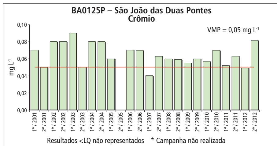
Gráfico 5.15.5 – Série histórica das concentrações de cromo no ponto BA0125P – São João das Duas Pontes, Aquífero Bauru
