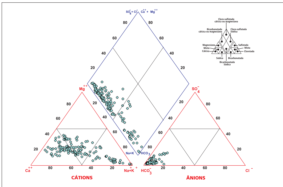
Figura 4.1.1 – Classificação das águas do Aquífero Bauru, segundo o Diagrama de Piper
