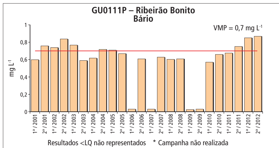
Gráfico 5.10.5 – Série histórica das concentrações de bário no ponto GU0111P – Ribeirão Bonito, Aquífero Guarani
