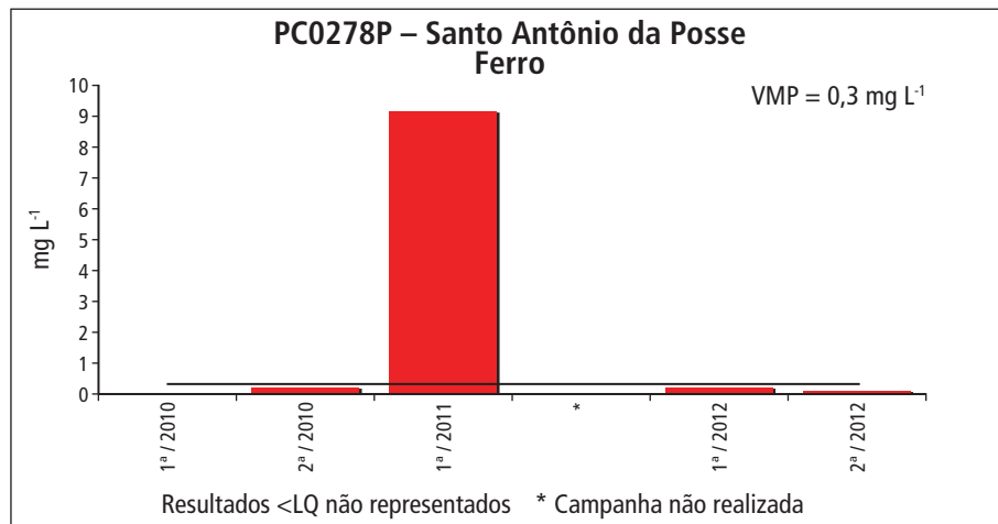
Gráfico 5.3.3 – Série histórica dos resultados para ferro no ponto PC0278P – Santo Antonio de Posse, Aquífero Pré-Cambriano
