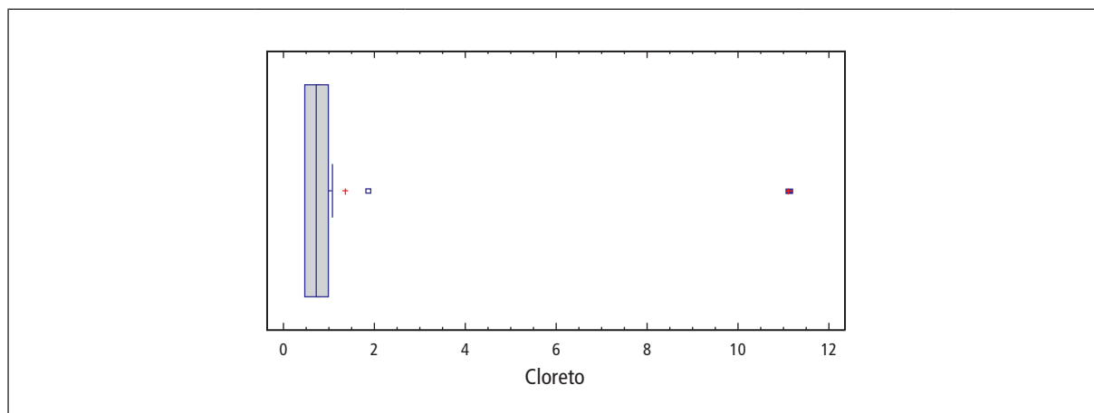
Gráfico 6.8 – Boxplot das concentrações de Cloreto ( \text{mg L}^{-1} ) das amostras de água subterrânea do Aquífero Guarani no período de 2010 a 2012
