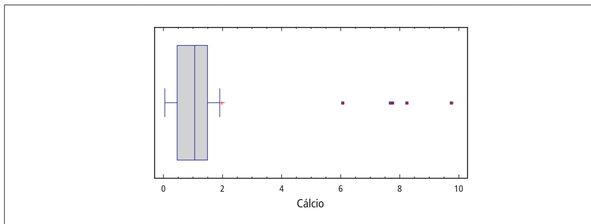
Gráfico 6.9 – Boxplot das concentrações de Cálcio ( \text{mg L}^{-1} ) das amostras de água subterrânea do Aquífero Guarani no período de 2010 a 2012
