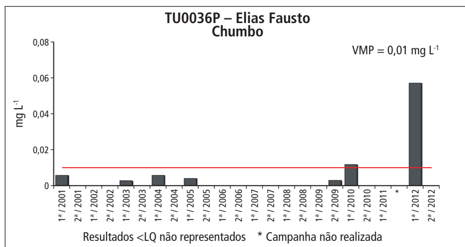
Gráfico 5.3.4 – Série histórica das concentrações de chumbo no ponto TU0036P – Elias Fausto, Aquífero Tubarão
