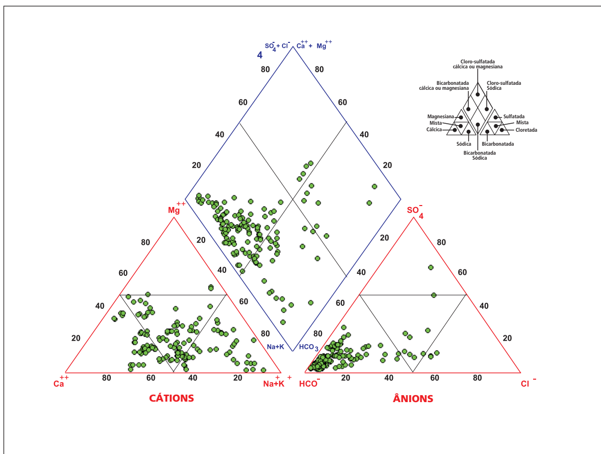
Figura 4.5.1 – Classificação das águas do Aquífero Pré-Cambriano, segundo o Diagrama de Piper
