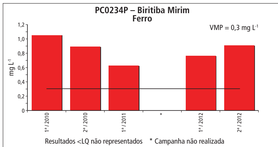
Gráfico 5.4.2 – Série histórica das concentrações de ferro no ponto PC0234P – Biritiba Mirim, Aquífero Pré-Cambriano
