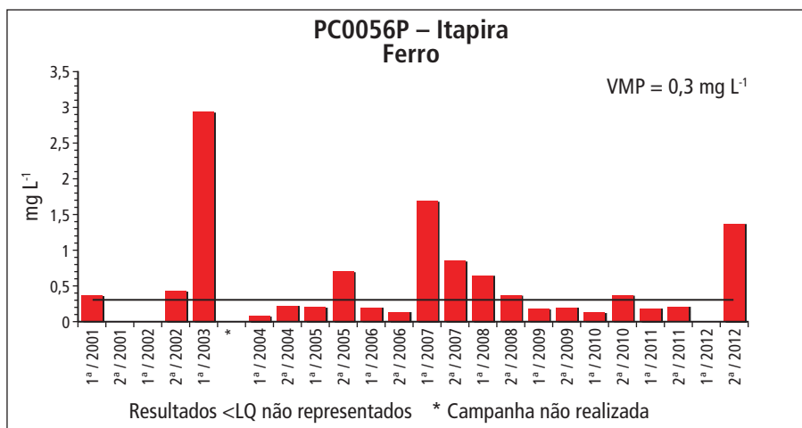
Gráfico 5.6.2 – Série histórica das concentrações de ferro no ponto PC0056P – Itapira, Aquífero Pré-Cambriano
