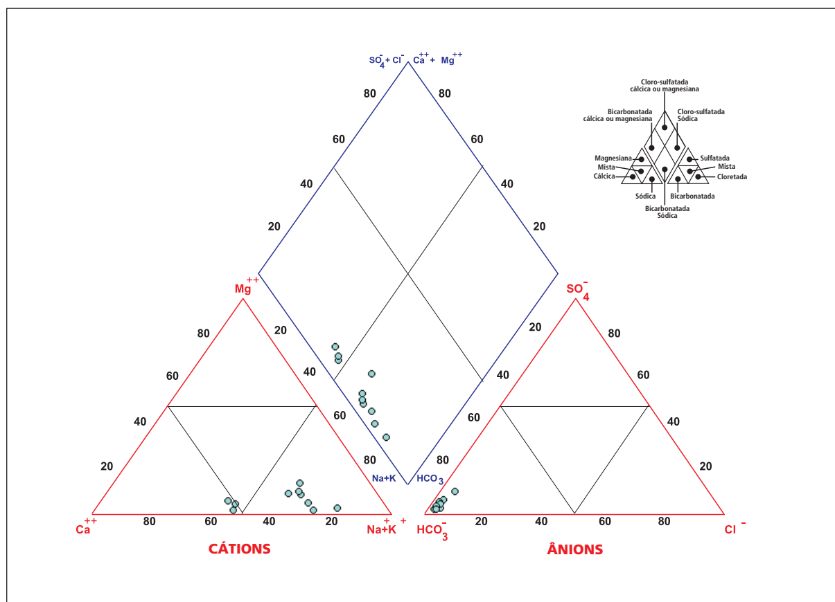
Figura 4.6.1 – Classificação das águas subterrâneas do Aquífero Taubaté, segundo o Diagrama de Piper
