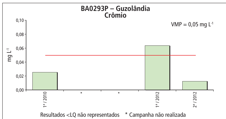
Gráfico 5.15.7 – Série histórica das concentrações de cromo no ponto BA0293P – Guzolândia, Aquífero Bauru
