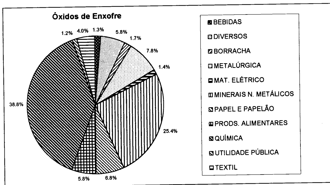
Gráfico 4 - Emissão de SO x por atividade industrial
