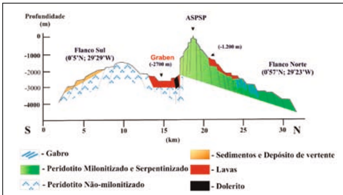
Figura 2.5. Perfil geológico interpretativo dos flancos norte e sul da cadeia transversal do ASPSP, que estão separados por uma falha transformante ativa de direção EW (HEKINIAN et al. , 2000).
