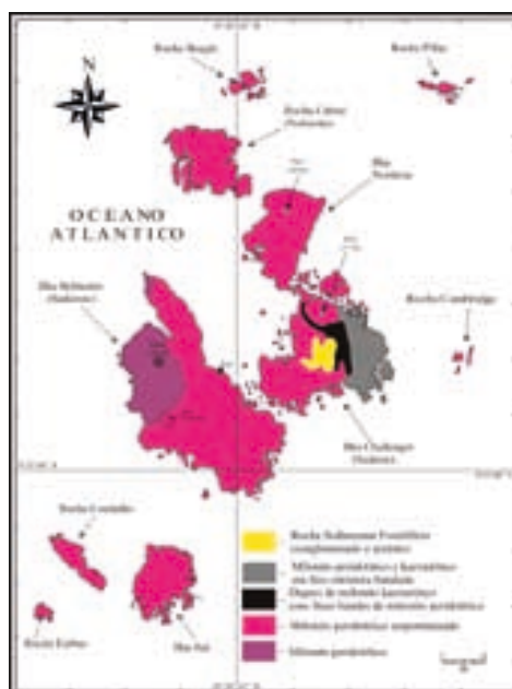
Figura 2.6. Mapa geológico da área emergida do Arquipélago de São Pedro e São Paulo, Atlântico equatorial (CAMPOS et al. , 2002, 2003a,b,c, 2004a,b,c,d, 2005a,b,c).
