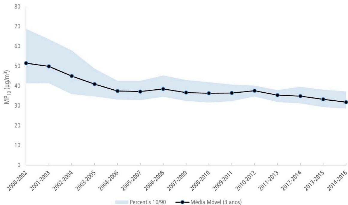
Gráfico 11 – MP_{10} – Evolução das médias móveis das médias anuais – RMSP.
