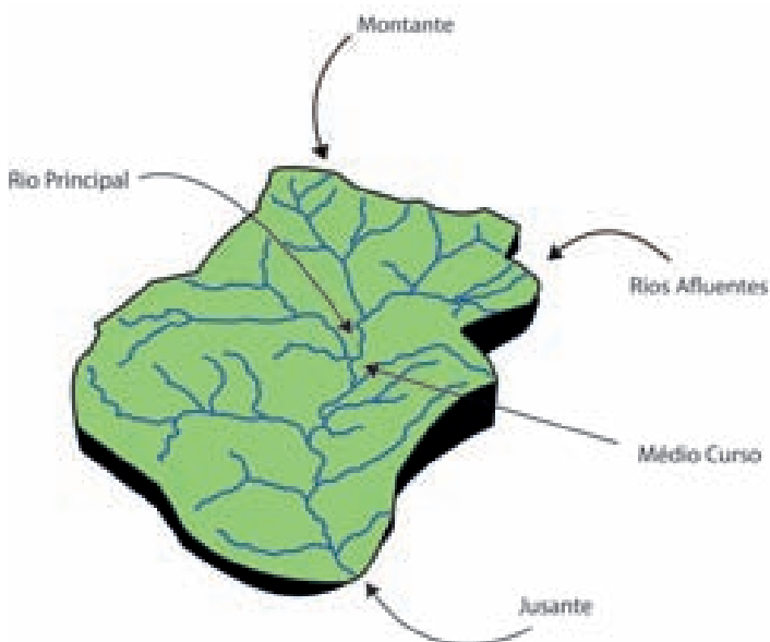
Representação de Bacia Hidrográfica
