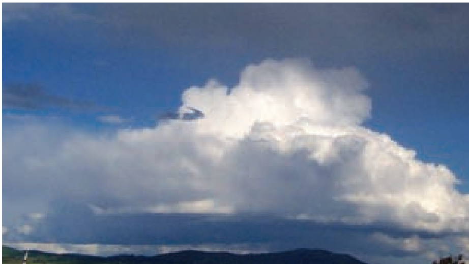
Cúmulo-nimbo (Maio de 2005). Foto: Fir 0002.
