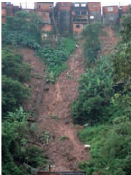
Escorregamento ameaça estabilidade das moradias no topo e na base da encosta em São Bernardo do Campo (Janeiro de 2010). Foto: Acervo IG.
