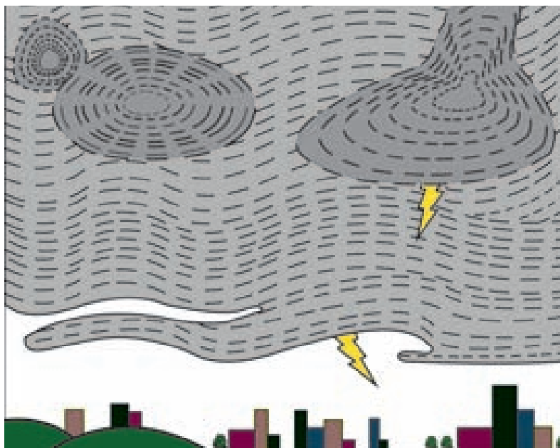
Formação de tempestade com ocorrência de raios sobre cidade.
