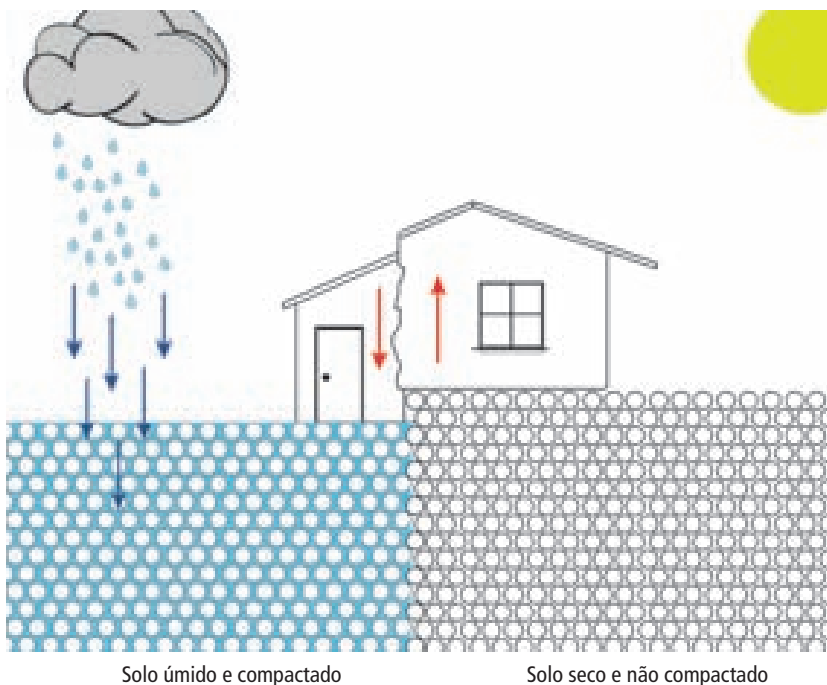
Subsidência em área urbana.
