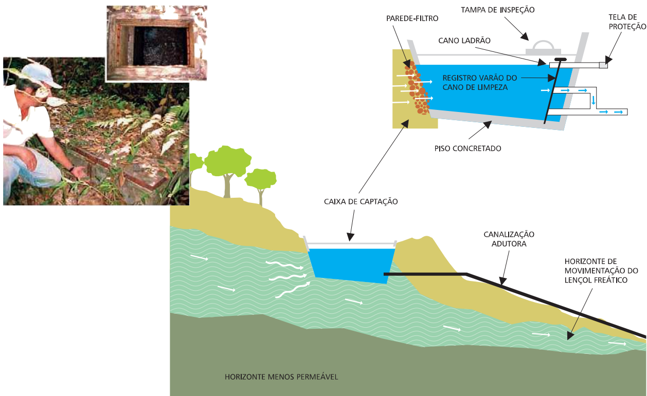
Figura 15. Caixa de proteção de nascente tipo trincheira.
