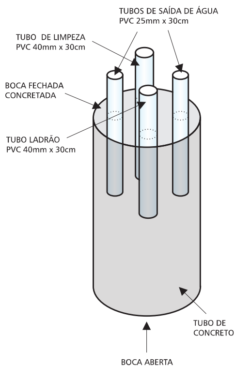
Figura 17. Proteção de fonte modelo Caxambu.
