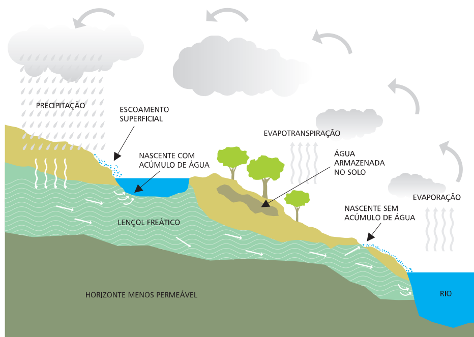
Figura 1. Ciclo hidrológico
