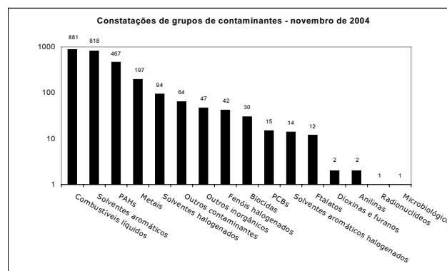
Figura 4.9 - Principais grupos de contaminantes constatados nas áreas contaminadas. Fonte: Cetesb.
