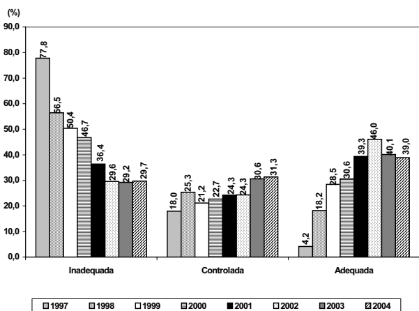
Figura 4.5 – Distribuição dos municípios do Estado de São Paulo quanto à qualidade dos aterros de resíduos domiciliares – Período 1997 a 2004. Fonte: Cetesb, 2005.
