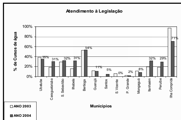
Figura 2.13 - Comparação dos índices de atendimento à legislação em 2003 e 2004. Fonte: Cetesb, 2005 – Relatório de Qualidade das Águas Litorâneas no Estado de São Paulo – Balneabilidade das Praias 2004.
