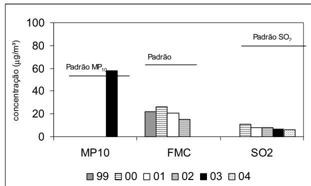
Figura 3.14. Evolução das concentrações médias anuais dos poluentes em Jundiá no período 1999-2004. Fonte: Cetesb, 2005 - Relatório de Qualidade do Ar no Estado de São Paulo
