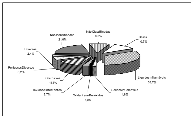
Figura 6.20 – Distribuição de acidentes com produtos químicos por classe de risco para o período de 1978 a 2004. Fonte: Cetesb.
