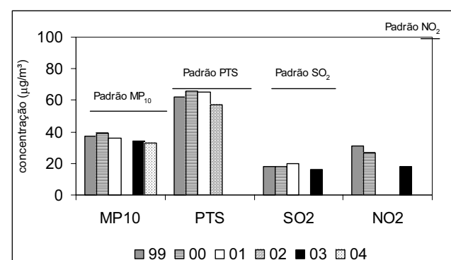
Figura 3.7. Evolução das concentrações médias anuais dos poluentes em Cubatão – Centro, no período 1999-2004. Fonte: Cetesb, 2005 – Relatório de Qualidade do Ar no Estado de São Paulo.
