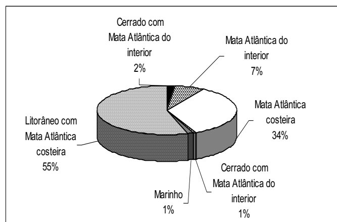
Figura 5.2. Distribuição percentual da área abrangida pelas unidades de conservação de proteção integral por biomas e ecorregiões. Fonte: Instituto Florestal.
