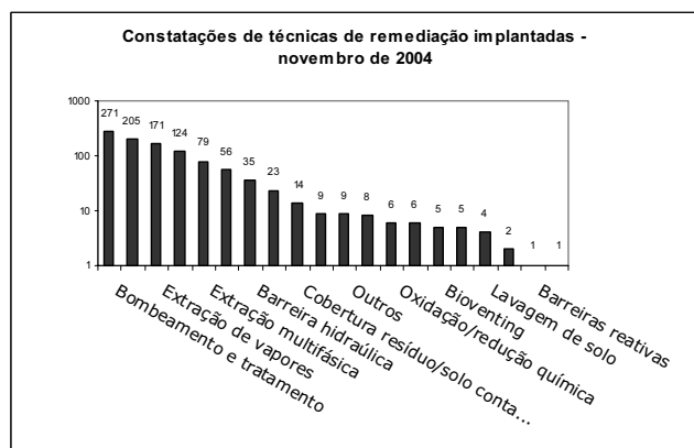
Figura 4.11 – Relação das técnicas de remediação implantadas nos casos constatados de áreas contaminadas. Fonte: Cetesb.
