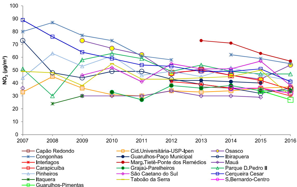
Gráfico 31 – NO 2 – Evolução das concentrações médias – RMSF (Rede Automática - maio a setembro)
