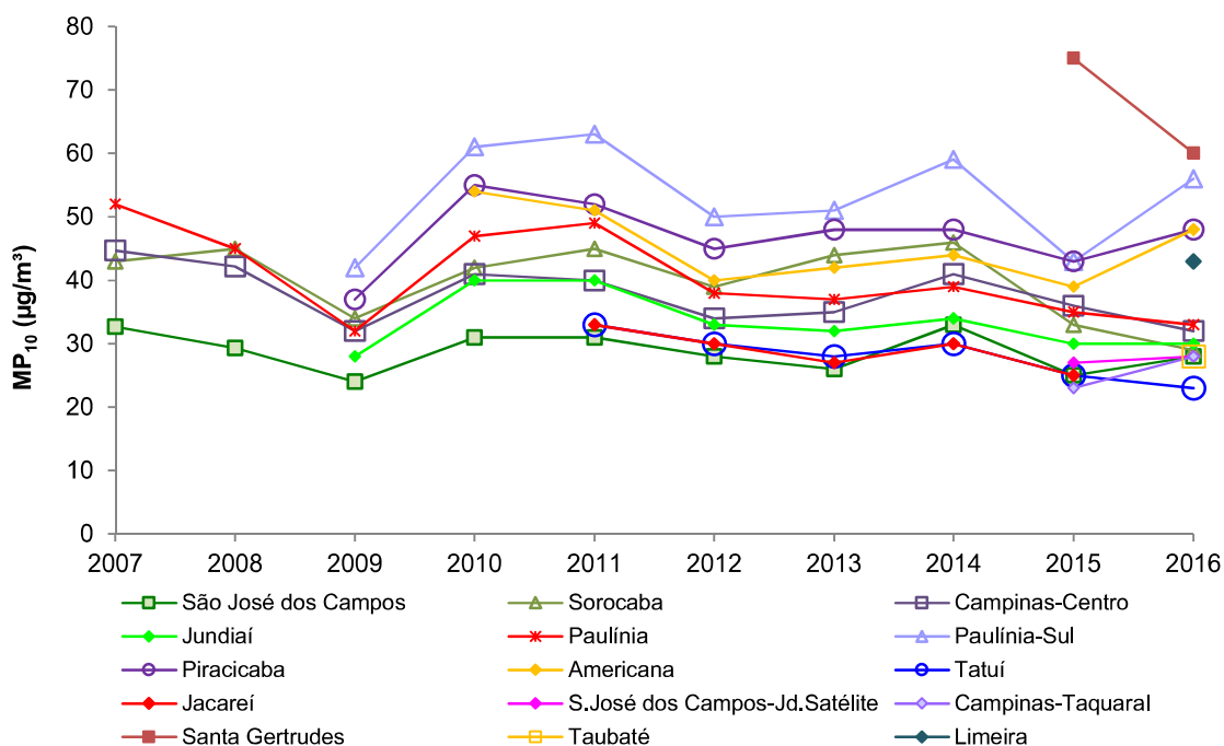
Gráfico 19 – MP 10 – Evolução das concentrações médias – UGRHs 2, 5 e 10 (Rede Automática - maio a setembro)
