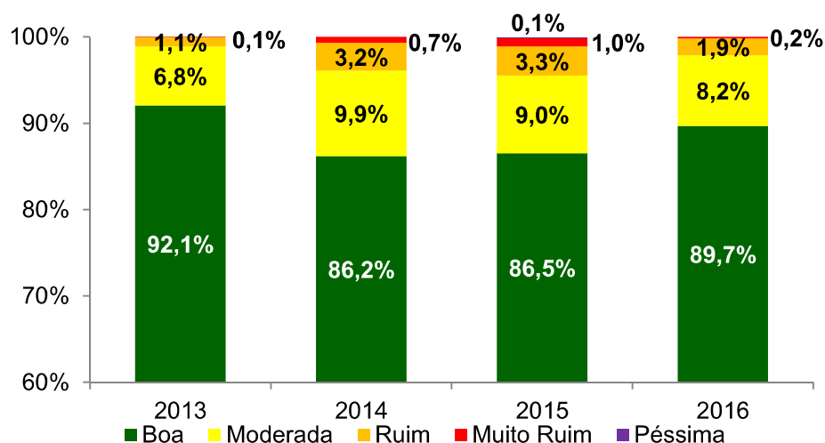
Gráfico 32 – O 3 – Distribuição percentual da qualidade do ar – RMSP (Rede Automática - janeiro a setembro)
