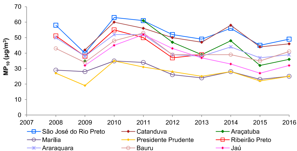
Gráfico 20 – MP 10 – Evolução das concentrações médias – UGRHs 4, 13, 15, 21 e 22 (Rede Automática - maio a setembro)
