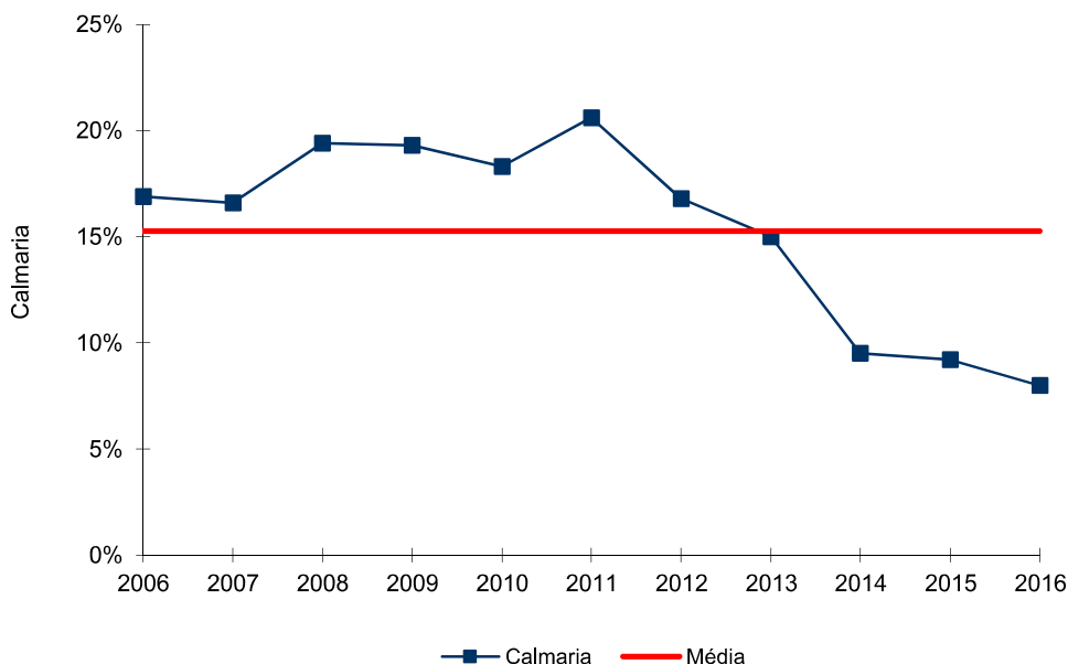
Gráfico 5 – Porcentagem de calmaria na RMSP CETESB – (maio a setembro)
