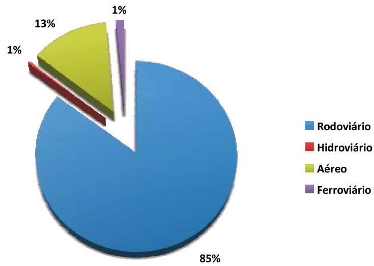
FIGURA 3.82 EMIÇÃO DE CO 2 NO SETOR DE TRANSPORTES NO ESTADO DE SÃO PAULO EM 2013
