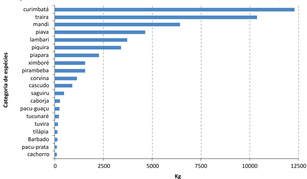
FIGURA 3.21 PRODUÇÃO DA PESCA EXTRATIVISTA MONITORADA PARA O RIO PARANAPANEMA (2003-2009)
