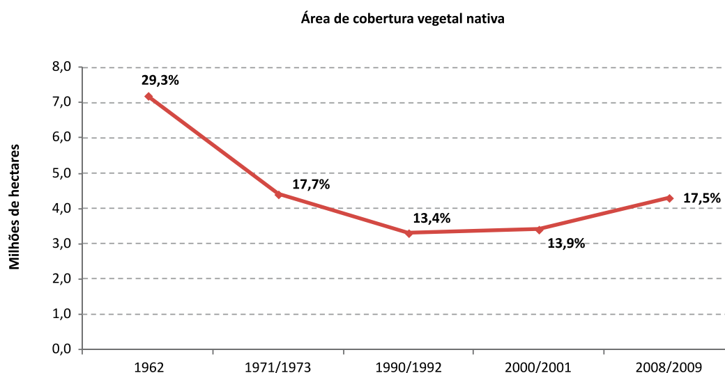
FIGURA 2.48 EVOLUÇÃO DA COBERTURA VEGETAL NATIVA NO ESTADO DE SÃO PAULO
