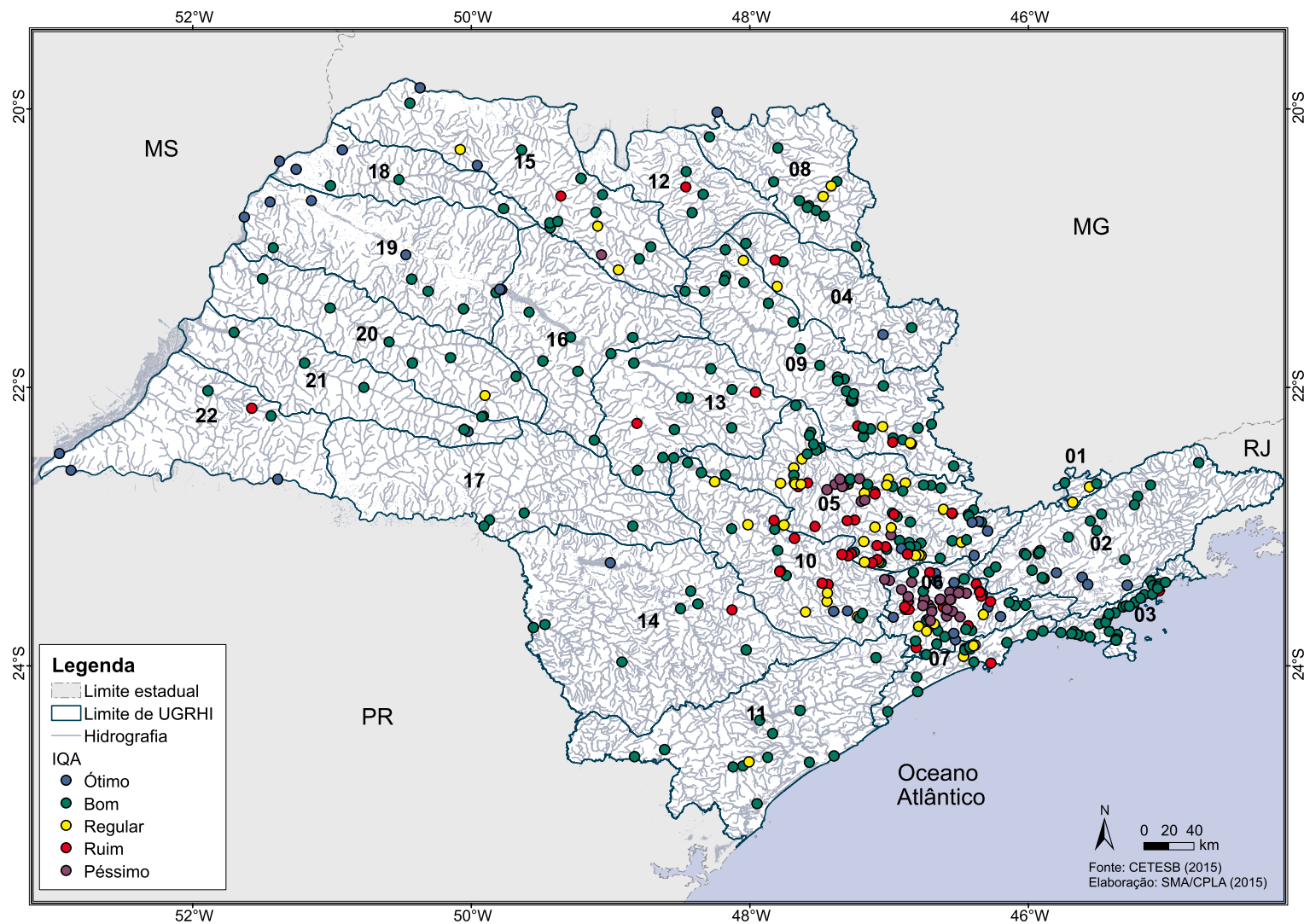
FIGURA 3.5 DISTRIBUIÇÃO DOS PONTOS DE MONITORAMENTO ENQUADRADOS NAS CLASSES DO ÍNDICE DE QUALIDADE DE ÁGUA (IQA) NO ESTADO DE SÃO PAULO EM 2014
