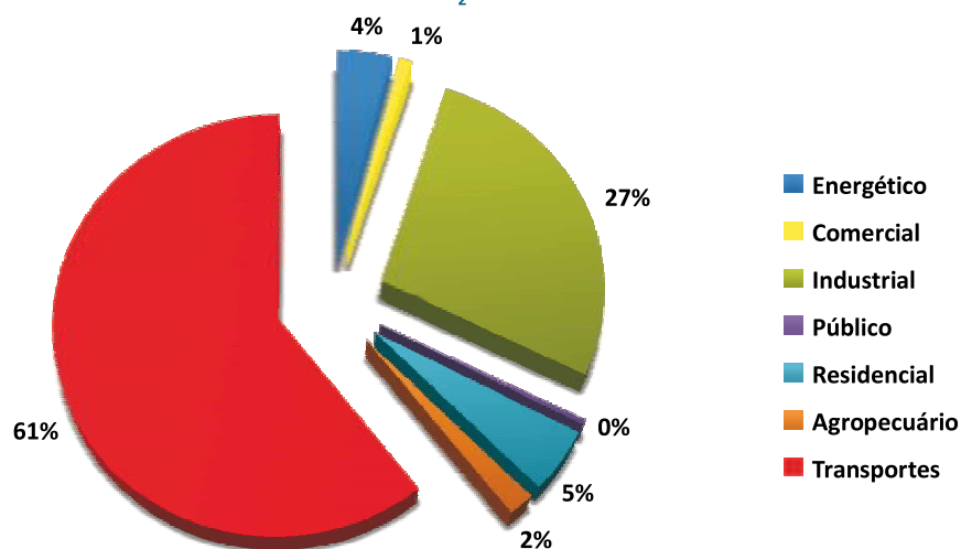
FIGURA 3.81 PARTICIPAÇÃO DOS SETORES NA EMISSÃO DE CO 2 DO ESTADO DE SÃO PAULO EM 2013
