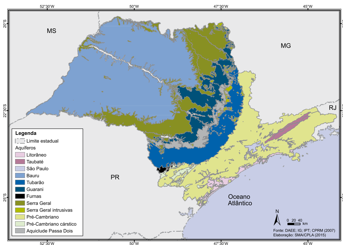
FIGURA 3.1 UNIDADES AQUIFERAS DO ESTADO DE SÃO PAULO
