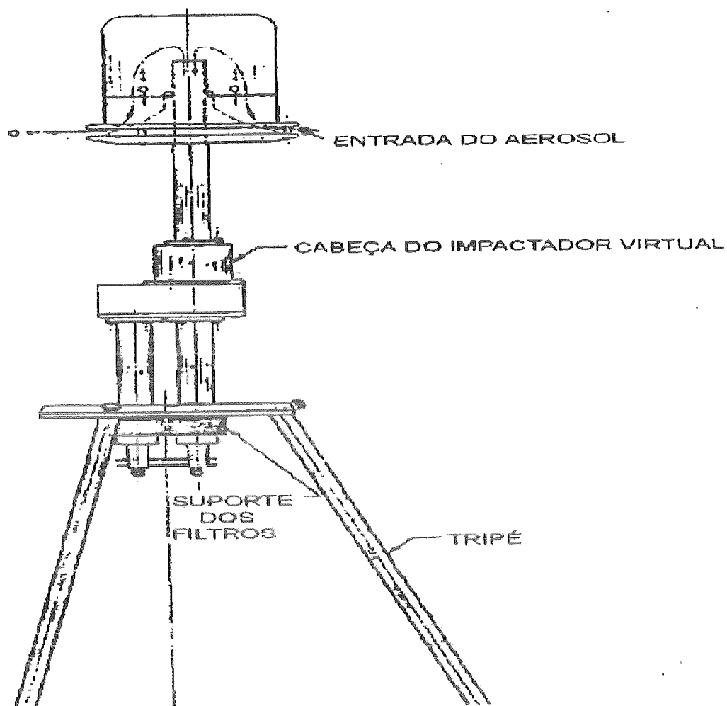
Figura 2 - Amostrador dicotômico
