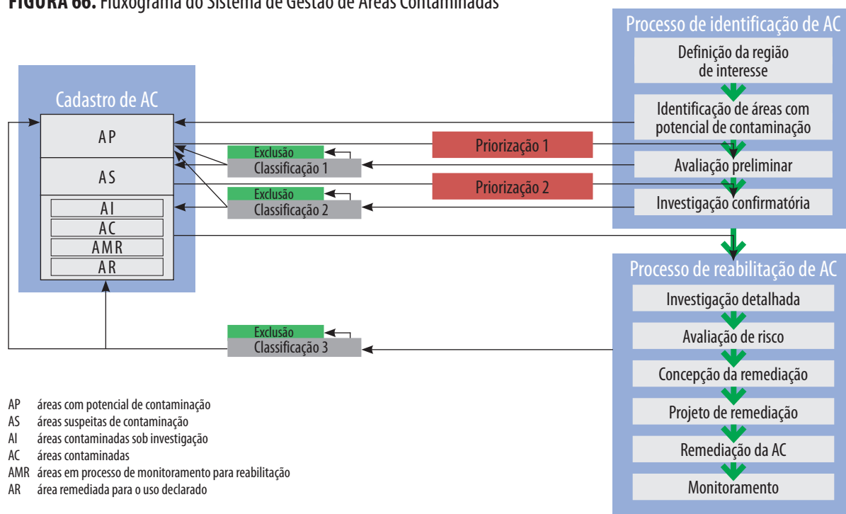
FIGURA 66. Fluxograma do Sistema de Gestão de Áreas Contaminadas
