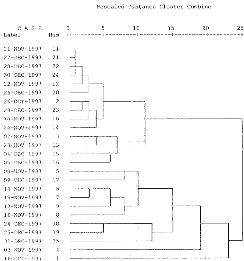
FIGURA 7 – Dendrograma representativo
