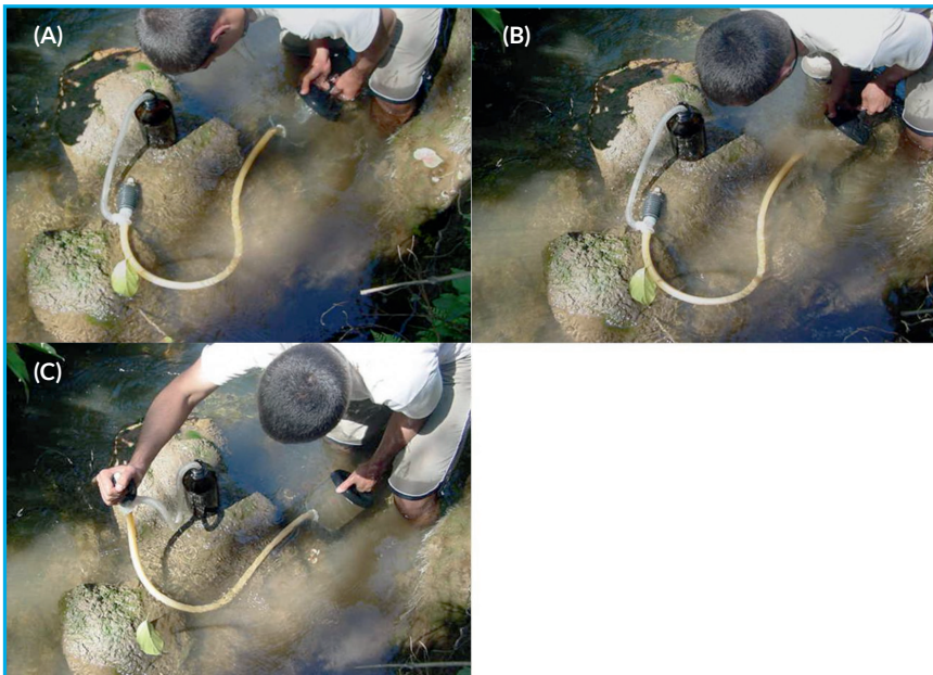
Figura 81. Coleta de amostras para Perífiton com perifitômetro com escova, modificado por VIS: (A) Introdução do amostrador no local selecionado, (B) Retirada do perífiton com a escova; (C) Bombeamento da água e perífiton raspado e preenchimento do frasco (Fotos: Rita Cerqueira Ribeiro de Souza/CETESB).
