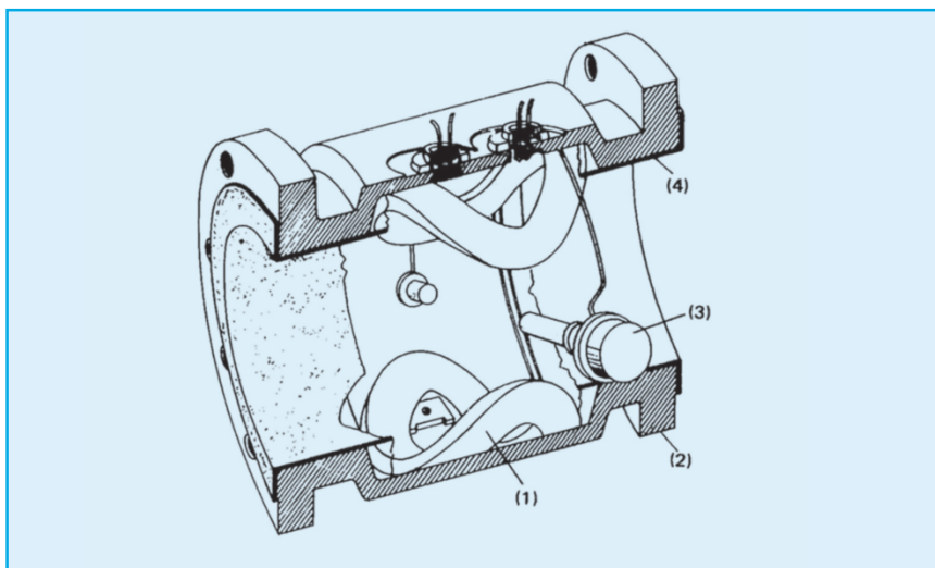
Figura 105. Medidor Magnético (Fonte: CETESB, 1988).
