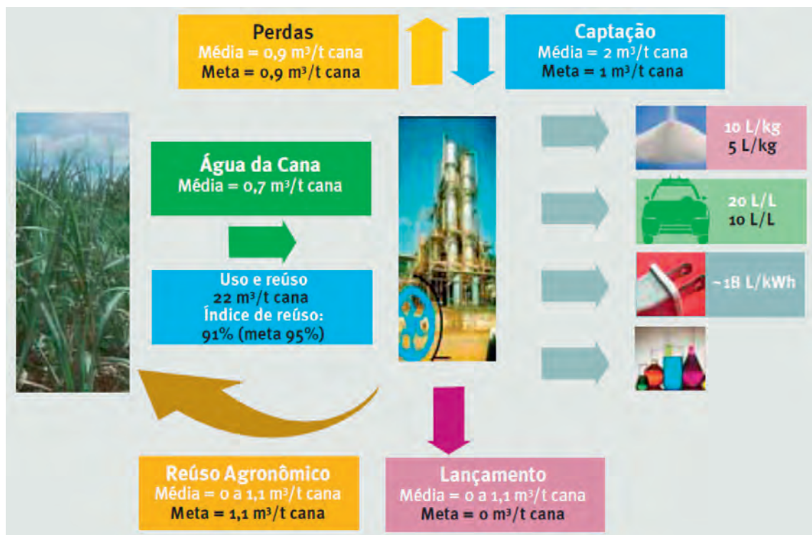
FIGURA 4. 2 BALANÇO MÉDIO GLOBAL DE ÁGUA NAS USINAS SUCROENERGÉTICAS
