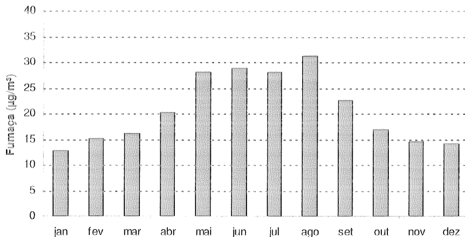
Figura 9 – Concentrações médias de fumaça por mês (1996-2005)
