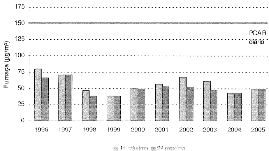
Figura 8 – Concentrações máximas de fumaça (1996-2005)
