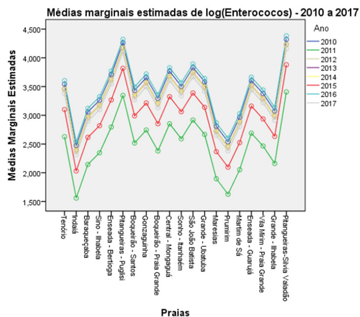
Gráfico 4.4 - Médias de enterococos por ano e praia (2010 a 2017)
