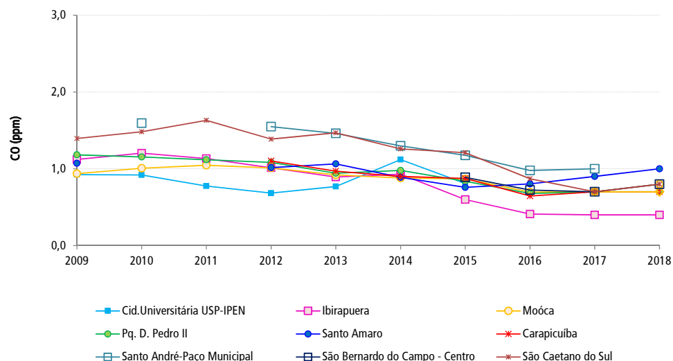
Gráfico 48 – CO – Evolução das médias anuais das concentrações máximas diárias (médias de 8 horas) – RMSP – Demais escalas
