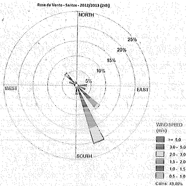
Figura 6 – Rosa de vento de Santos – 2012/2013 - 24h
