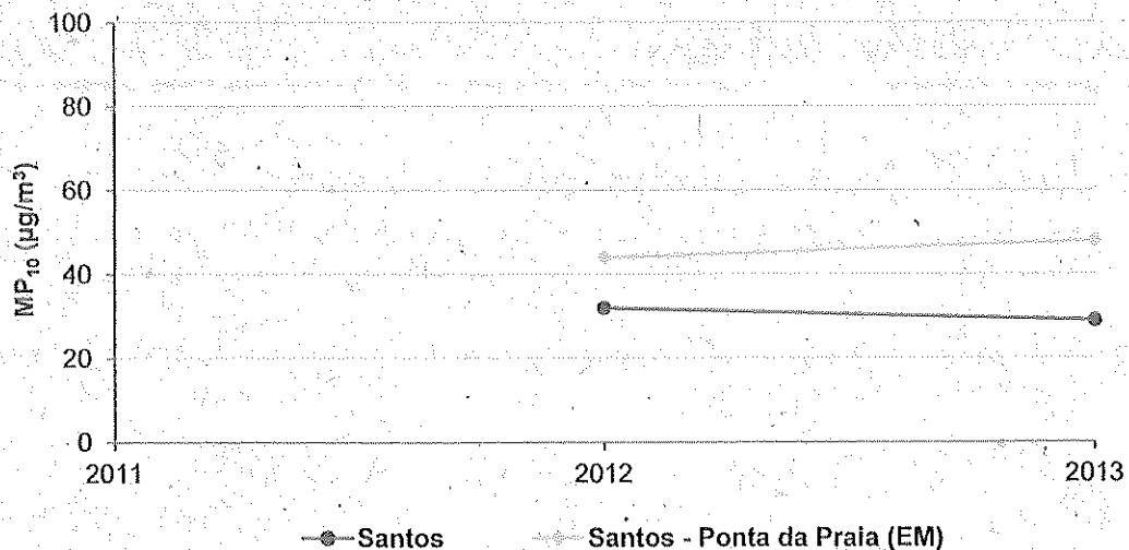
Gráfico 03 – MP_{10} - Evolução das concentrações médias anuais
