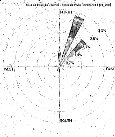
a) Rosa de poluição (1-6h)
