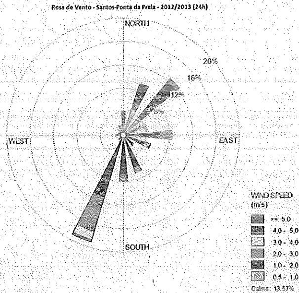
Figura 8 – Rosa de vento da Estação Santos-Ponta da Praia - EM – 2012/2013 - 24h
