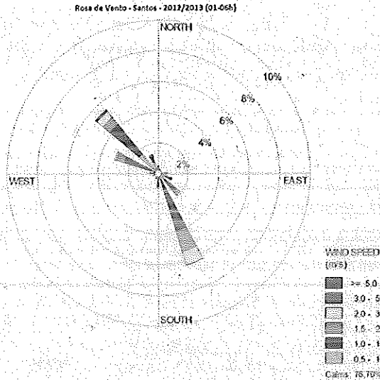
Figura 7-- Rosa de vento da Estação Santos, por período (1-6h, 7-12h, 13-18h, 19-24h)
