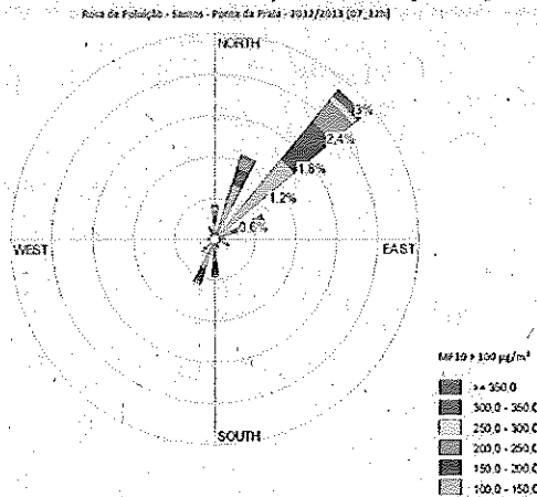
b) Rosa de poluição (7-12h)
