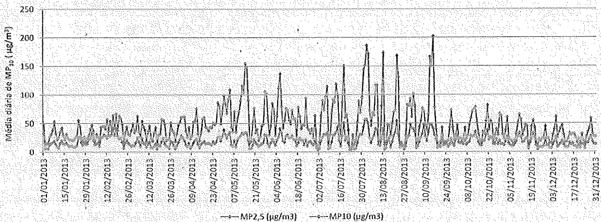
Gráfico 11 — Evolução das concentrações médias diárias de \text{MP}_{10} e \text{MP}_{2,5} – Santos-Ponta da Praia (EM)
