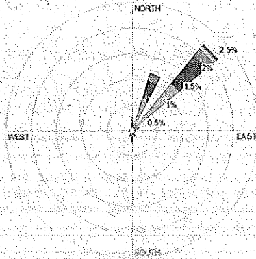
d) Rosa de poluição (19-24h)
