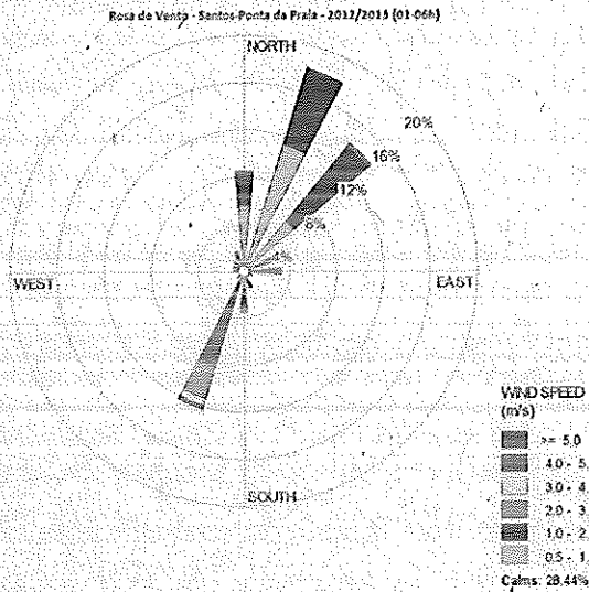
Figura 9 – Rosa de vento da Estação Móvel Santos-Ponta da Praia, por período (1-6h, 7-12h, 13-18h, 19-24h)
