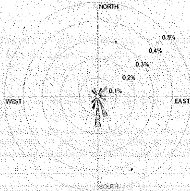
c) Rosa de poluição (13-18h)
