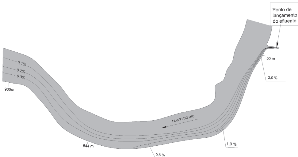
Figura 2 – Pluma de dispersão superficial de um efluente (isolinhas em %) no rio Paraíba do Sul
