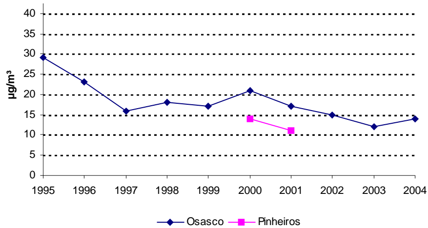
FIGURA 27 - SO 2 - Concentrações médias - Zona Oeste Período de maio a setembro
