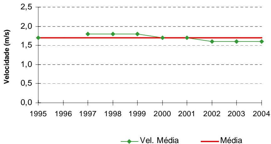
FIGURA 5 - Velocidade média do vento na Região Metropolitana de São Paulo Período maio a setembro (Rede Automática - CETESB)
