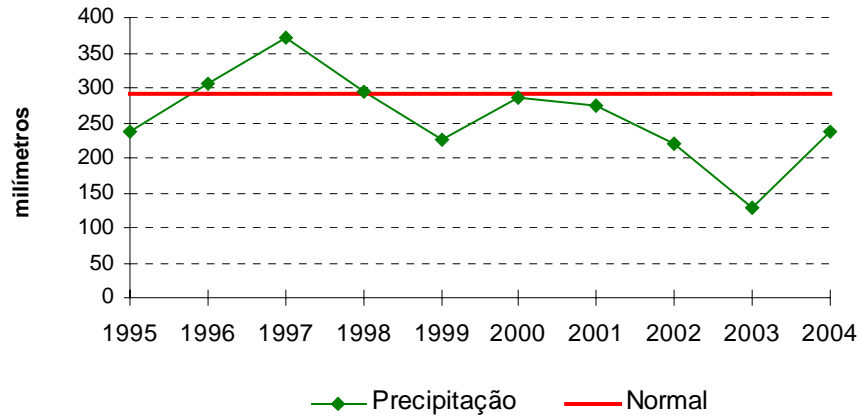
FIGURA 2 - Precipitação Total de 1995 a 2004 e Normal de 1961 a 1990 Período de maio a setembro (Estação Mirante de Santana - INMET)
