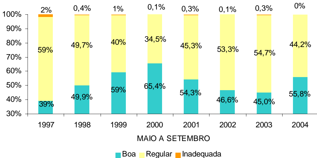
FIGURA 35 - NO 2 – Distribuição Percentual da Qualidade do Ar Período de maio a setembro
